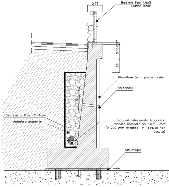
Figura 1: sezione tipologica del muro
