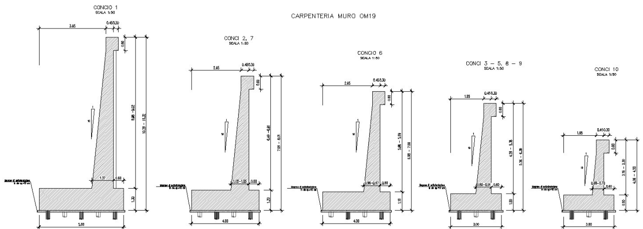
Figura 2: carpenteria del muro
