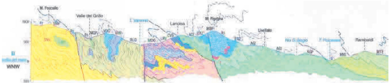
Figura 6-2 – Assetto geologico – Sezione geologica BB' da Foglio Genova n.213-230 della Carta Geologica d'Italia 1:50.000 (progetto CARG)
