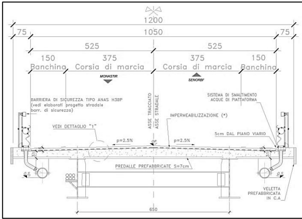
Figura 6. Sezione tipo C1 su viadotto.
