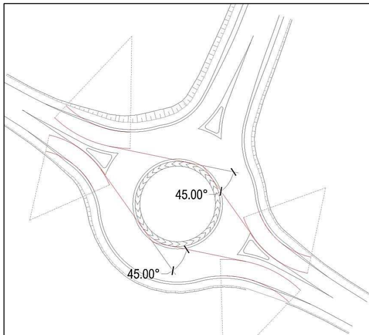
Figura 23 – Rotatoria ROT_BARRALI – Verifica delle traiettorie di deflessione.
