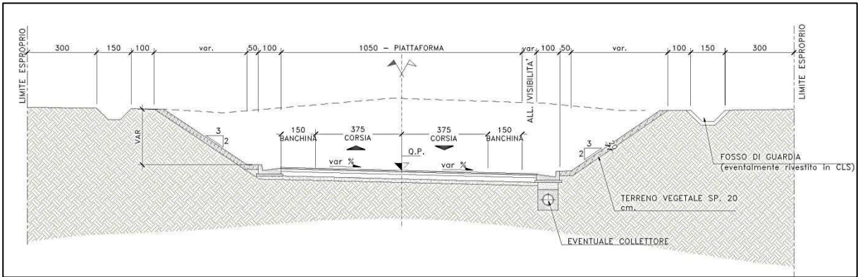
Figura 5. Sezione tipo C1 in trincea.
