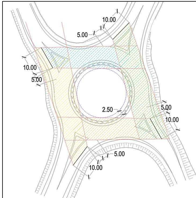
Figura 18 – Rotatoria ROT03 – Verifica delle visibilità a sinistra.
