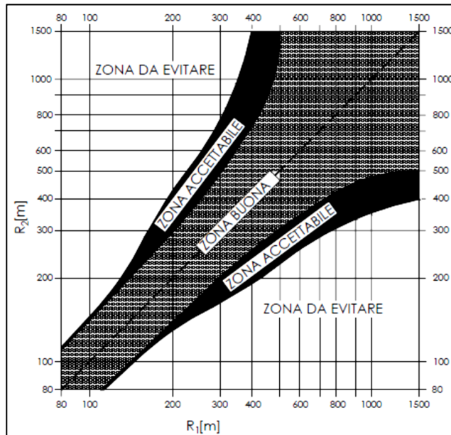
Figura 9. D.M. 05.11.2001 - Abaco figura 5.2.2.a.
