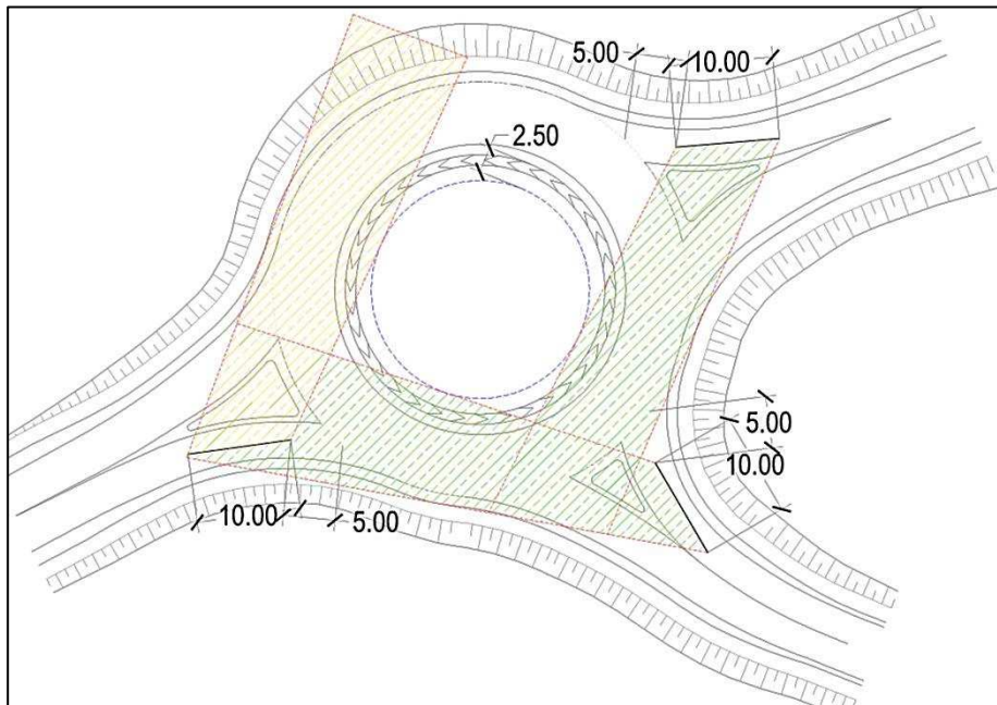
Figura 20 – Rotatoria ROT04 – Verifica delle visibilità a sinistra.
