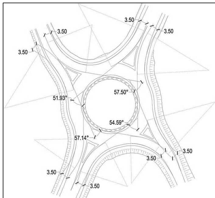
Figura 17 – Rotatoria ROT03 – Verifica delle traiettorie di deflessione.
