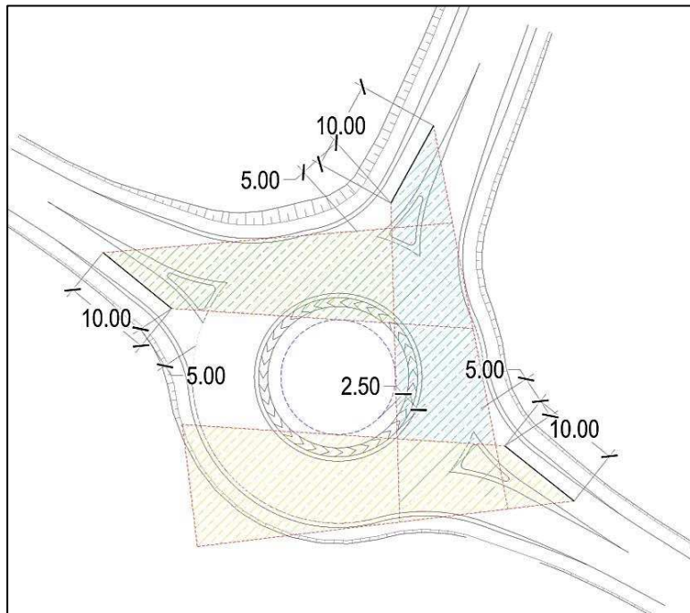
Figura 24 – Rotatoria ROT_BARRALI – Verifica delle visibilità a sinistra.
