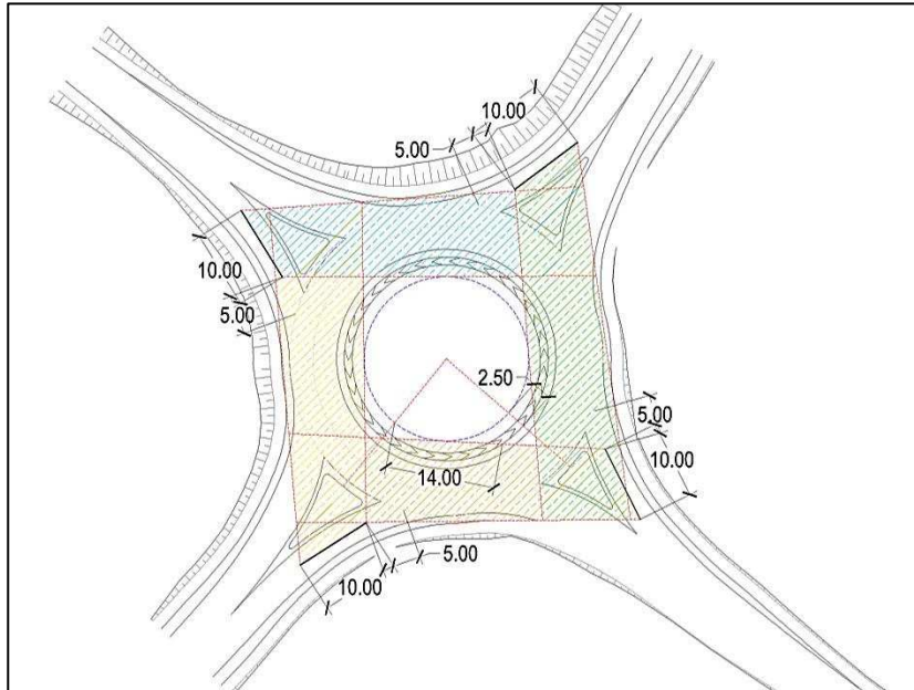
Figura 14 – Rotatoria ROT01 – Verifica delle visibilità a sinistra.
