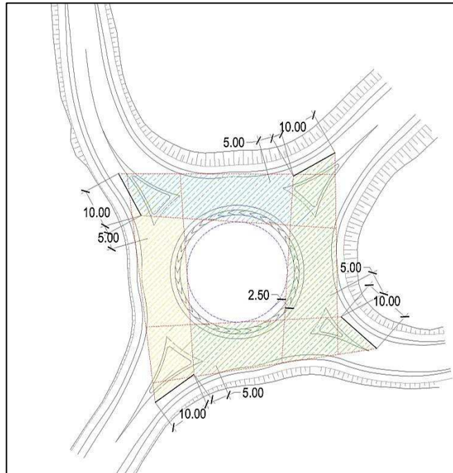
Figura 22 – Rotatoria ROT05 – Verifica delle visibilità a sinistra.
