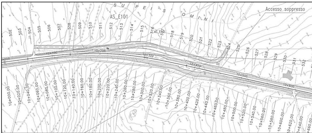
Figura 33. Viabilità AS_E101
