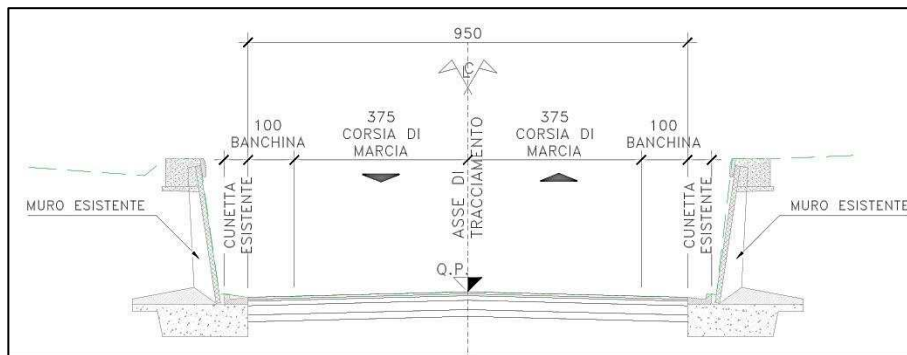
Figura 8. Sezione tipo tra muri esistenti
