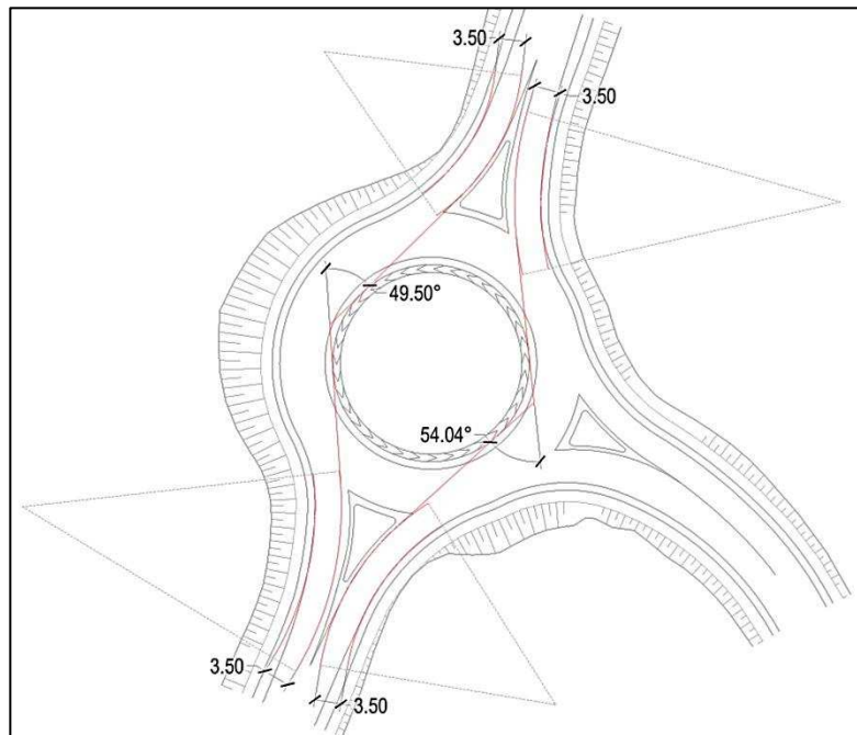
Figura 15 – Rotatoria ROT02 – Verifica delle traiettorie di deflessione.
