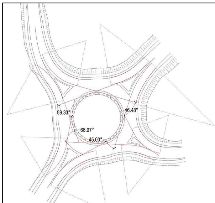
Figura 21 – Rotatoria ROT05 – Verifica delle traiettorie di deflessione.
