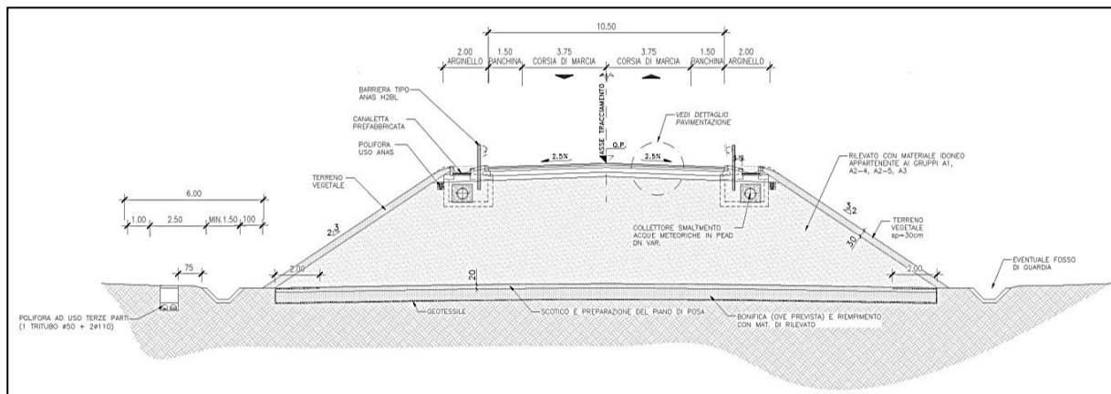
Figura 4. Sezione tipo C1 in rilevato.
