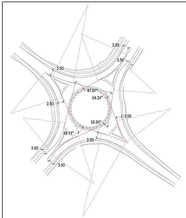
Figura 13 – Rotatoria ROT01 – Verifica delle traiettorie di deflessione.
