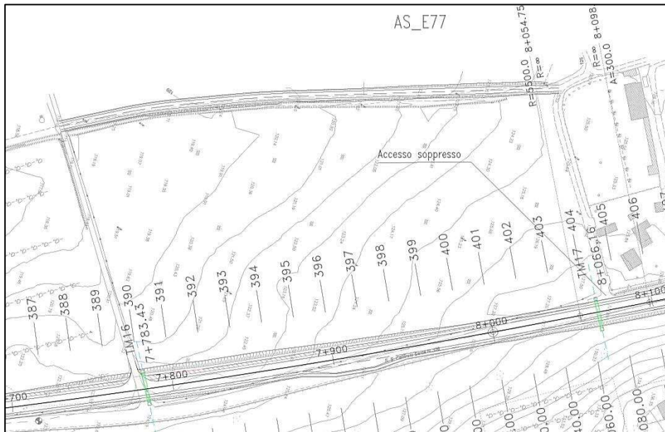
Figura 31. Viabilità AS_E77
