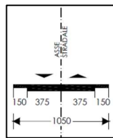
Figura 3. Piattaforma stradale tipo C1 (D.M. 05.11.2001).
