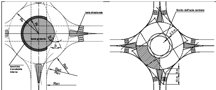
Figura 12. Schemi verifiche previste nel DM 19/04/2006.
