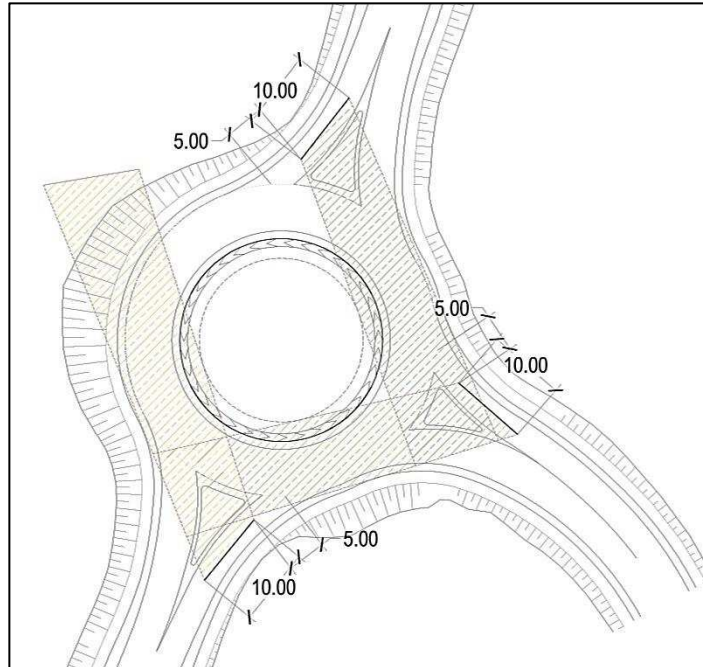
Figura 16 – Rotatoria ROT02 – Verifica delle visibilità a sinistra.
