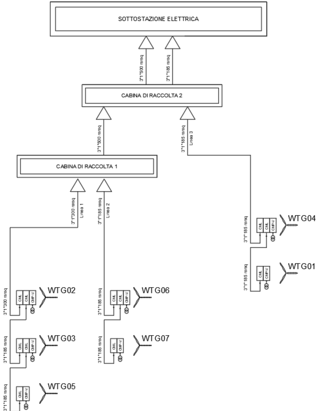
Schema Unifilare WTG
