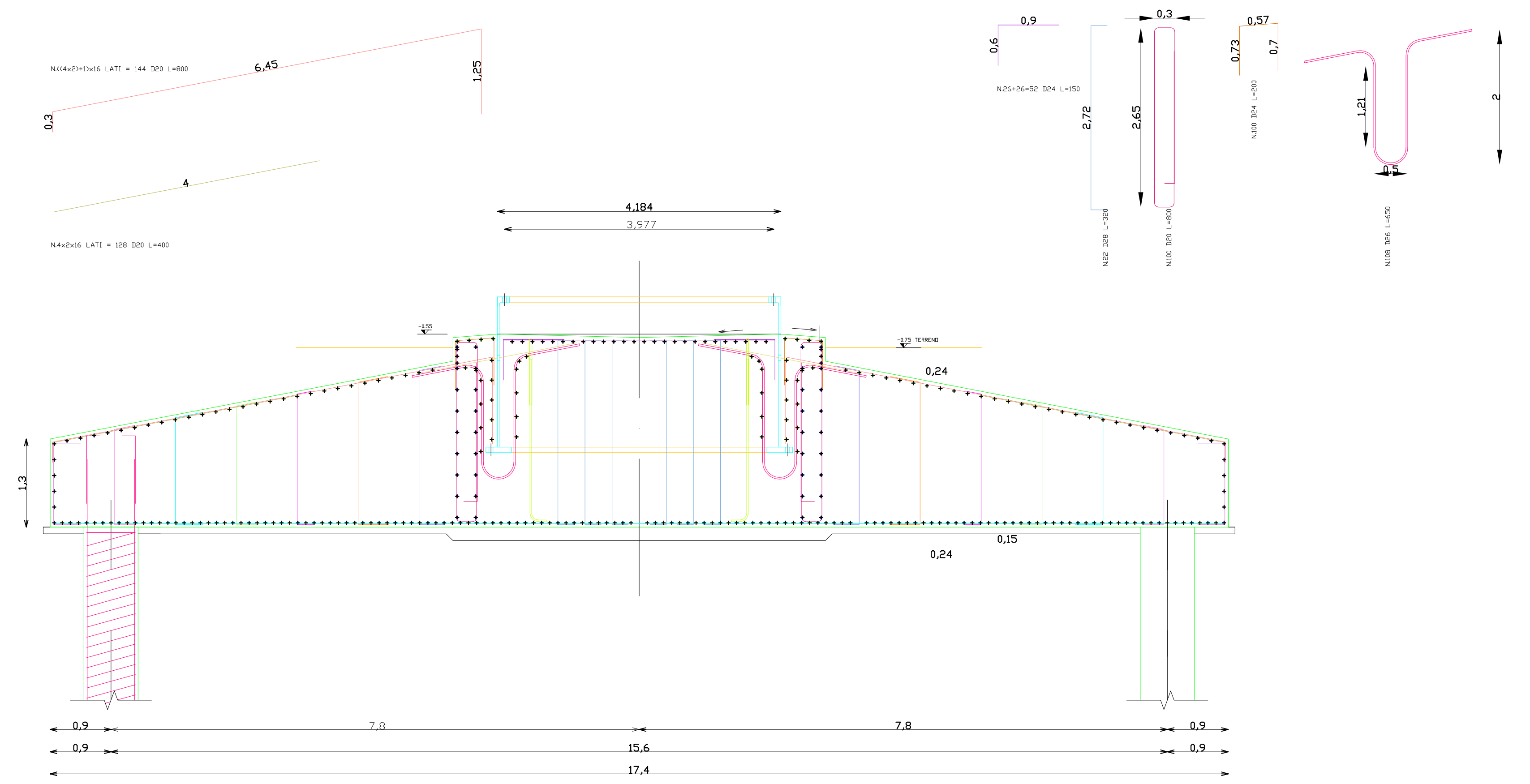
SEZIONE
