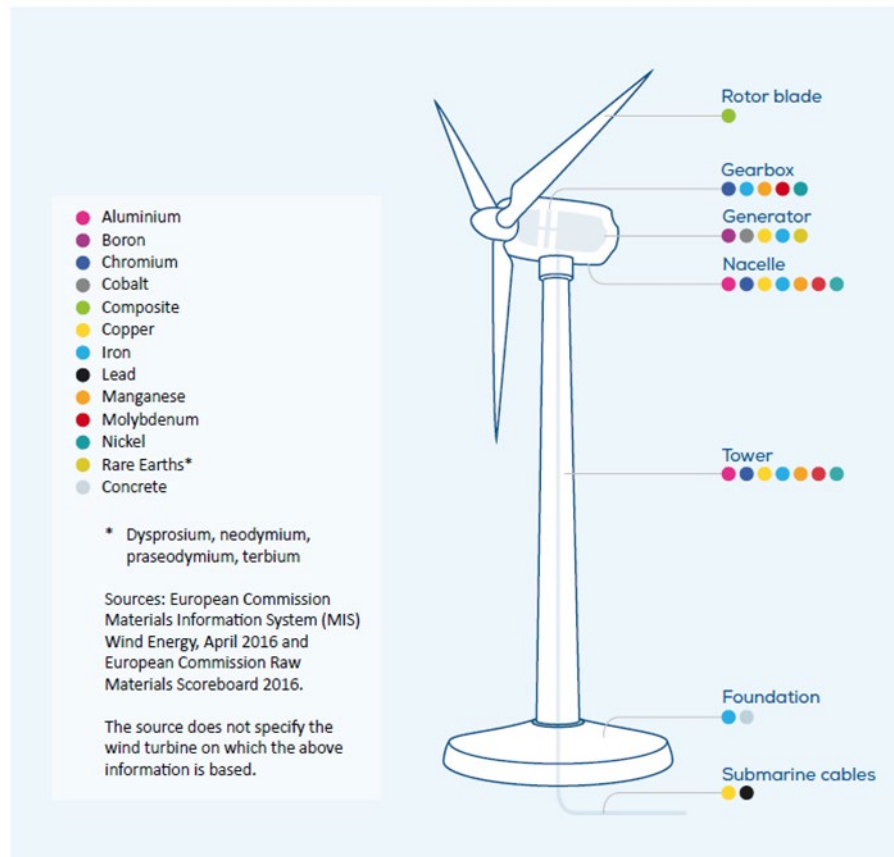
Figura 51: Indicazione dei materiali costituenti un aerogeneratore tipo
