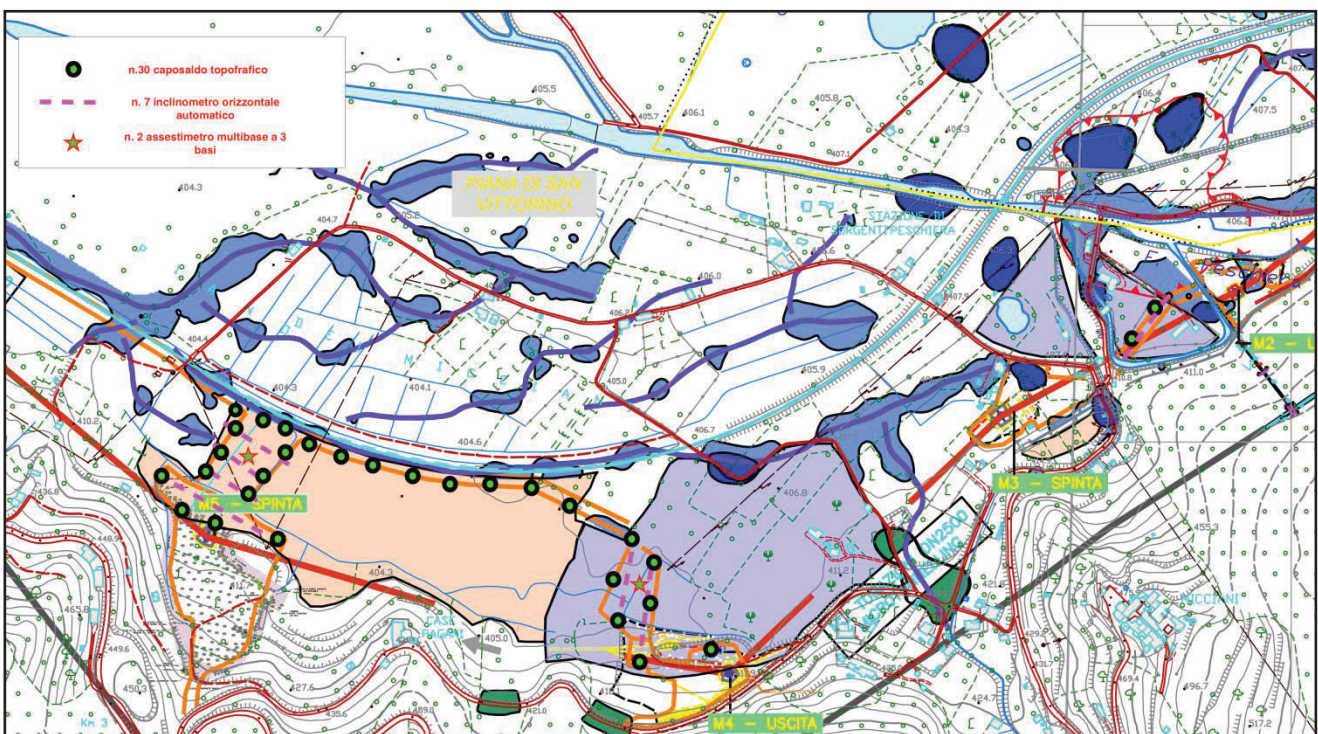
Esempio della distribuzione della sensoristica di monitoraggio nella piana di San Vittorino
