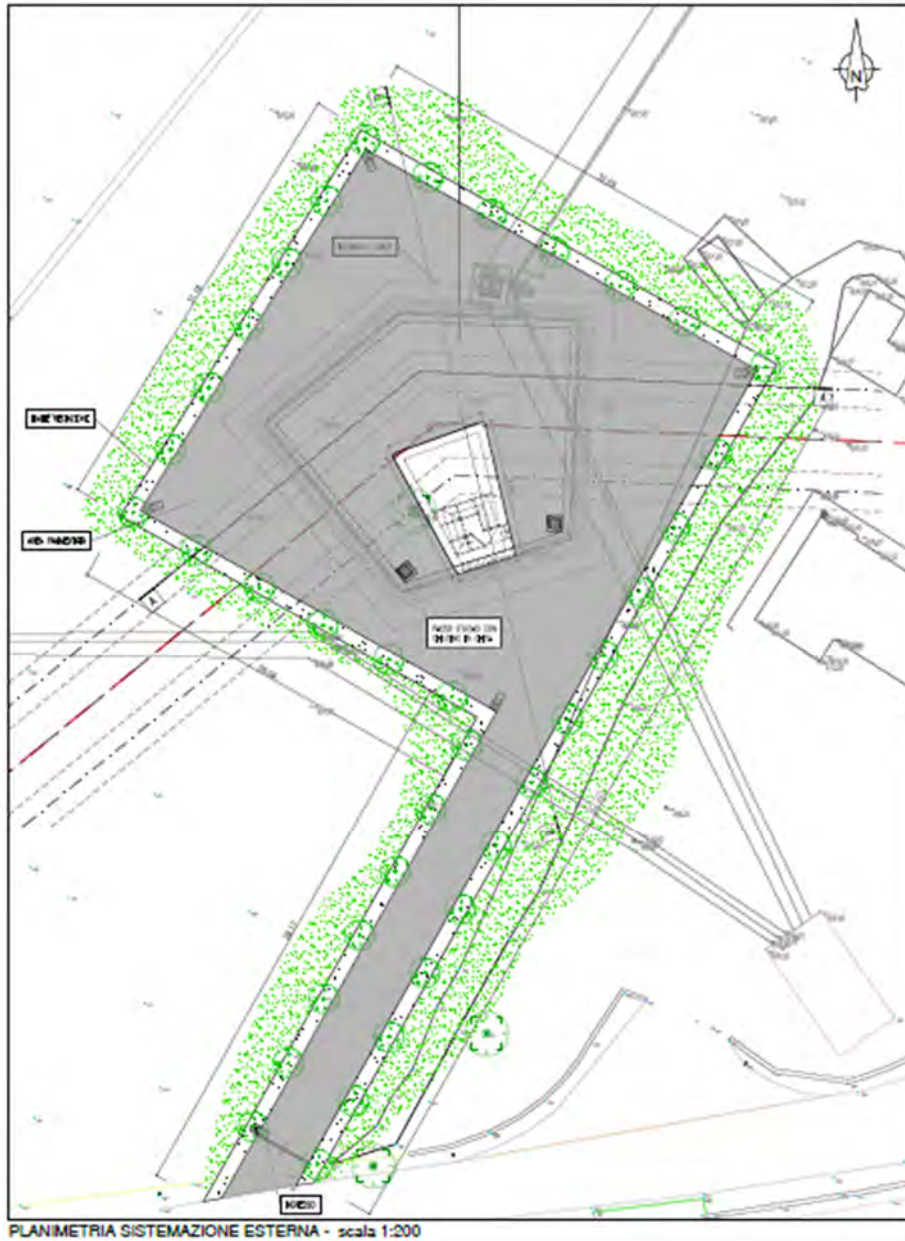
PLANIMETRIA SISTEMAZIONE ESTERNA - scala 1:200
