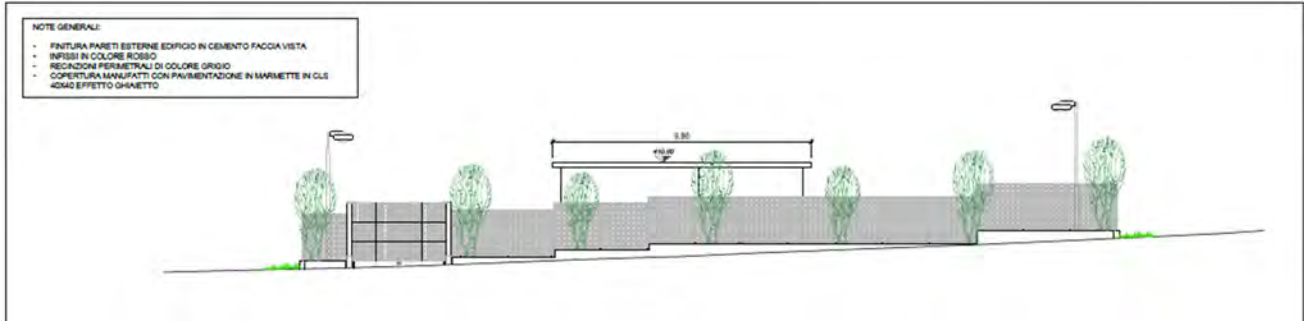
PROSPETTO SUD-OVEST - scala 1:100
