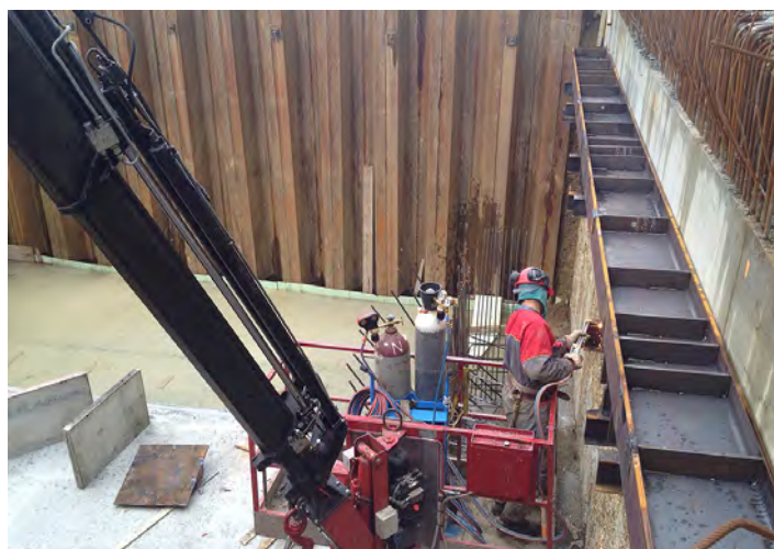
Figura 10.5 – Esempio realizzazione mensole e trave di ripartizione
