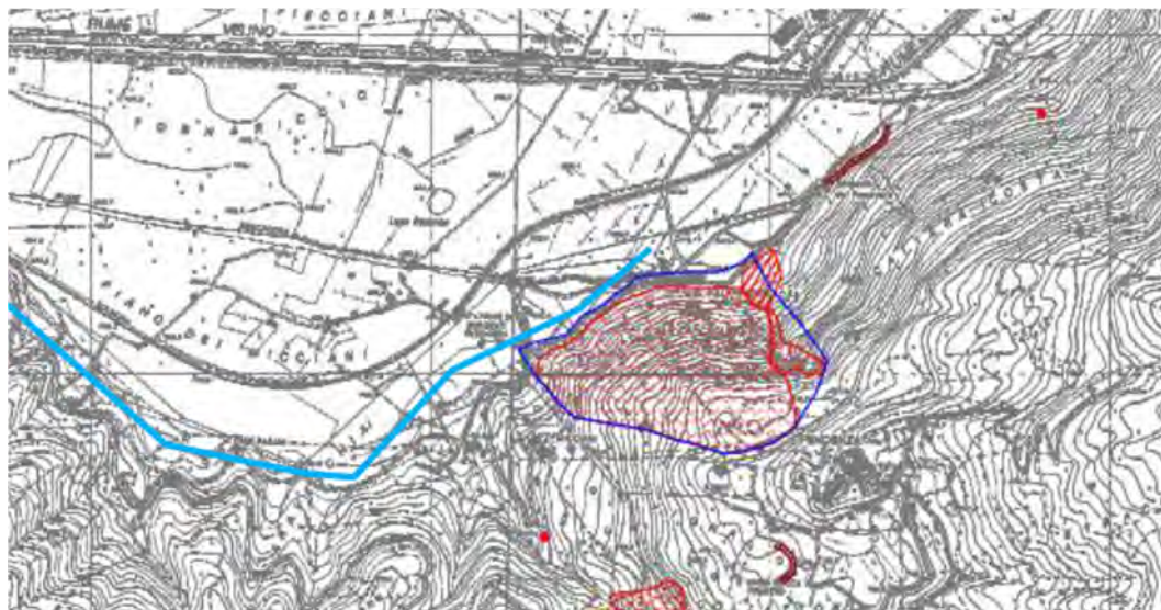
Figura 6.5 – Zone soggette ad instabilità gravitativa censite dal PAI nel settore in cui ricade il versante delle Sorgenti del Peschiera (DGPV). La linea azzurra rappresenta una porzione del tracciato di progetto.
