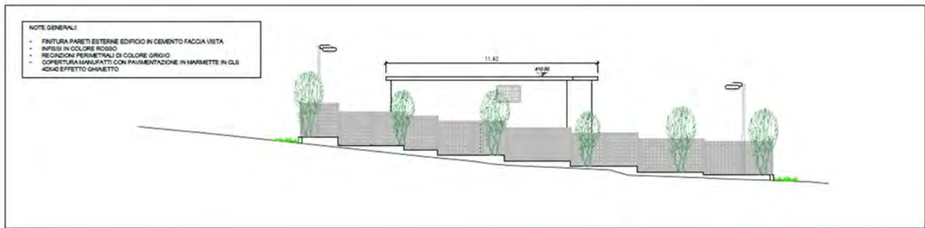
PROSPETTO SUD-EST - scala 1:100
