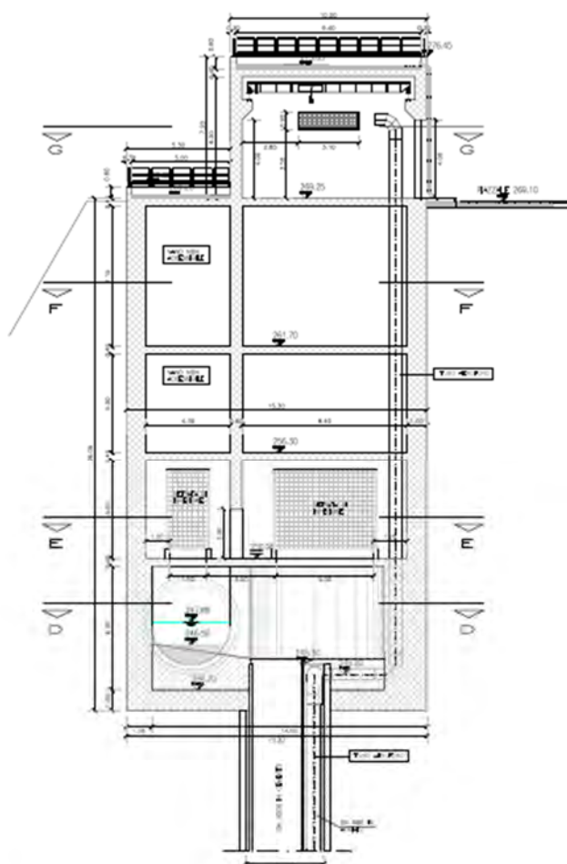
SEZIONE A - A - SCALA 1:100
