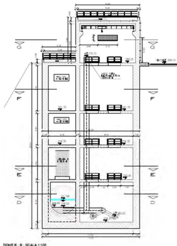
SEZIONE B - B - SCALA 1:100
