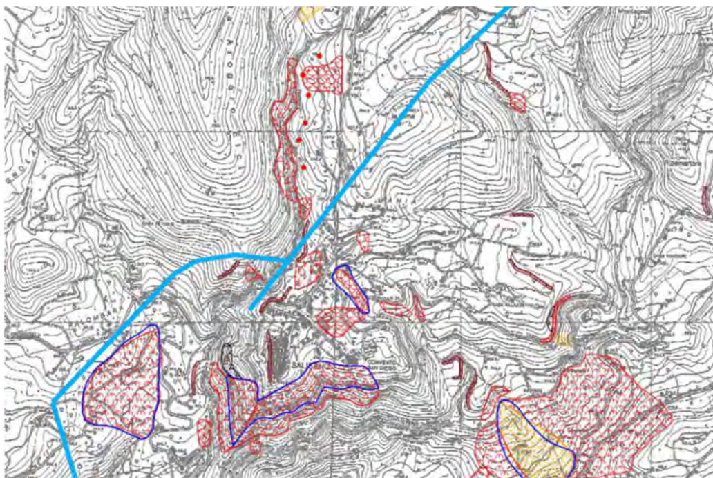
Figura 6.9 – Zone soggette ad instabilità gravitativa censite sia dal PAI presso l'abitato di Salisano. La linea azzurra rappresenta una porzione del tracciato di progetto.
