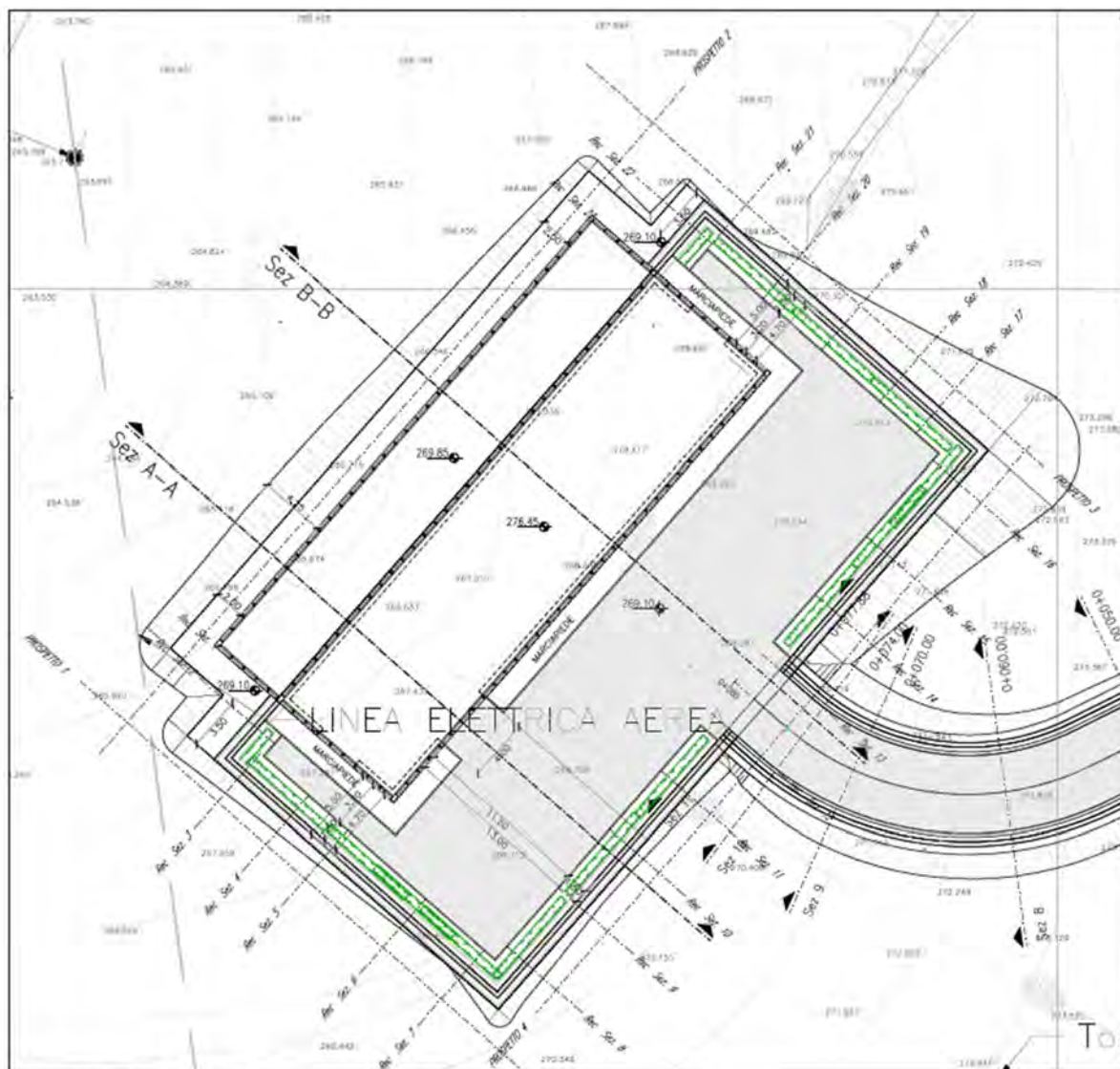
PLANIMETRIA GENERALE - SCALA 1:200
