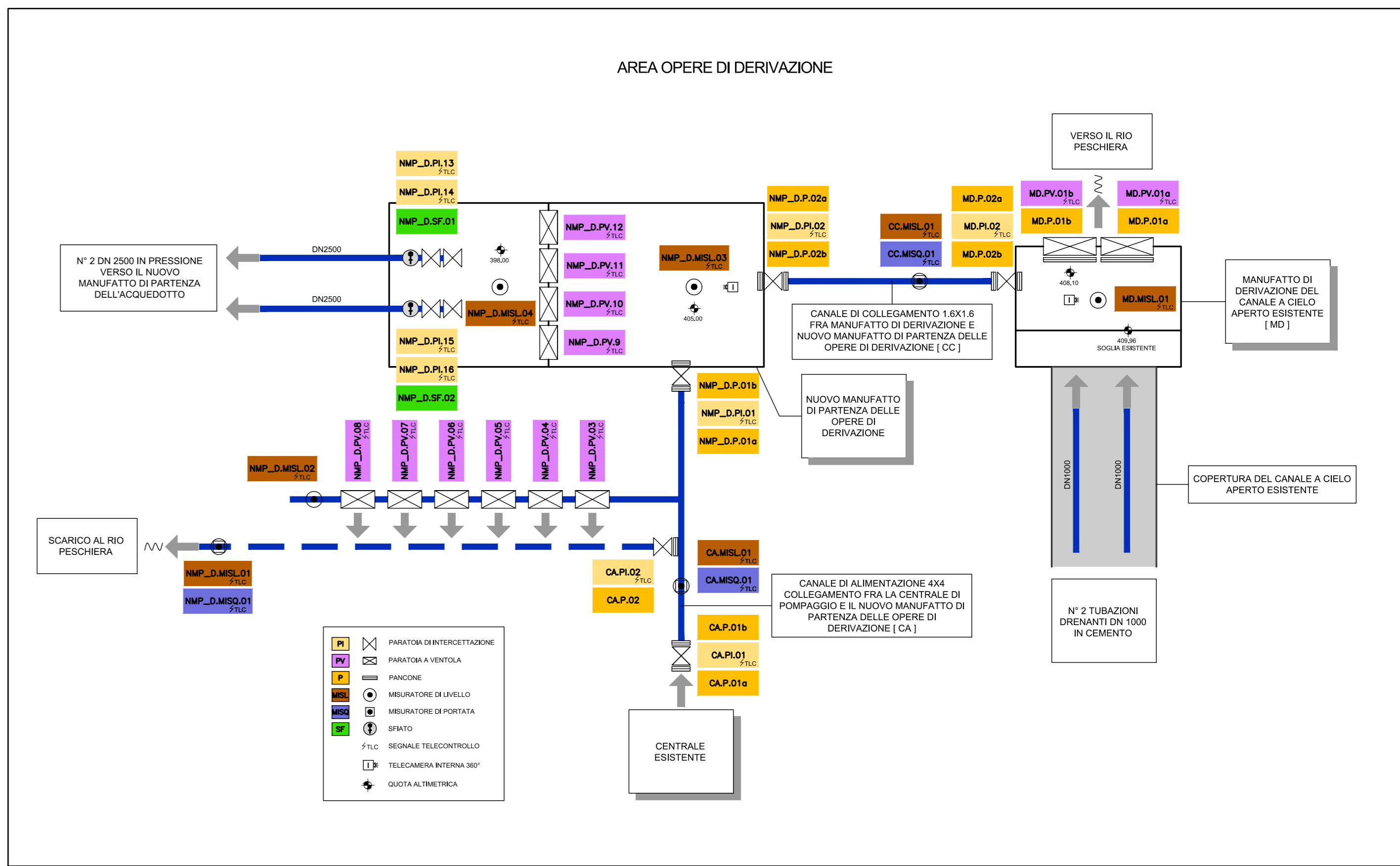
SCHEMA IDRAULICO FUNZIONALE - SCALA 1:2000
