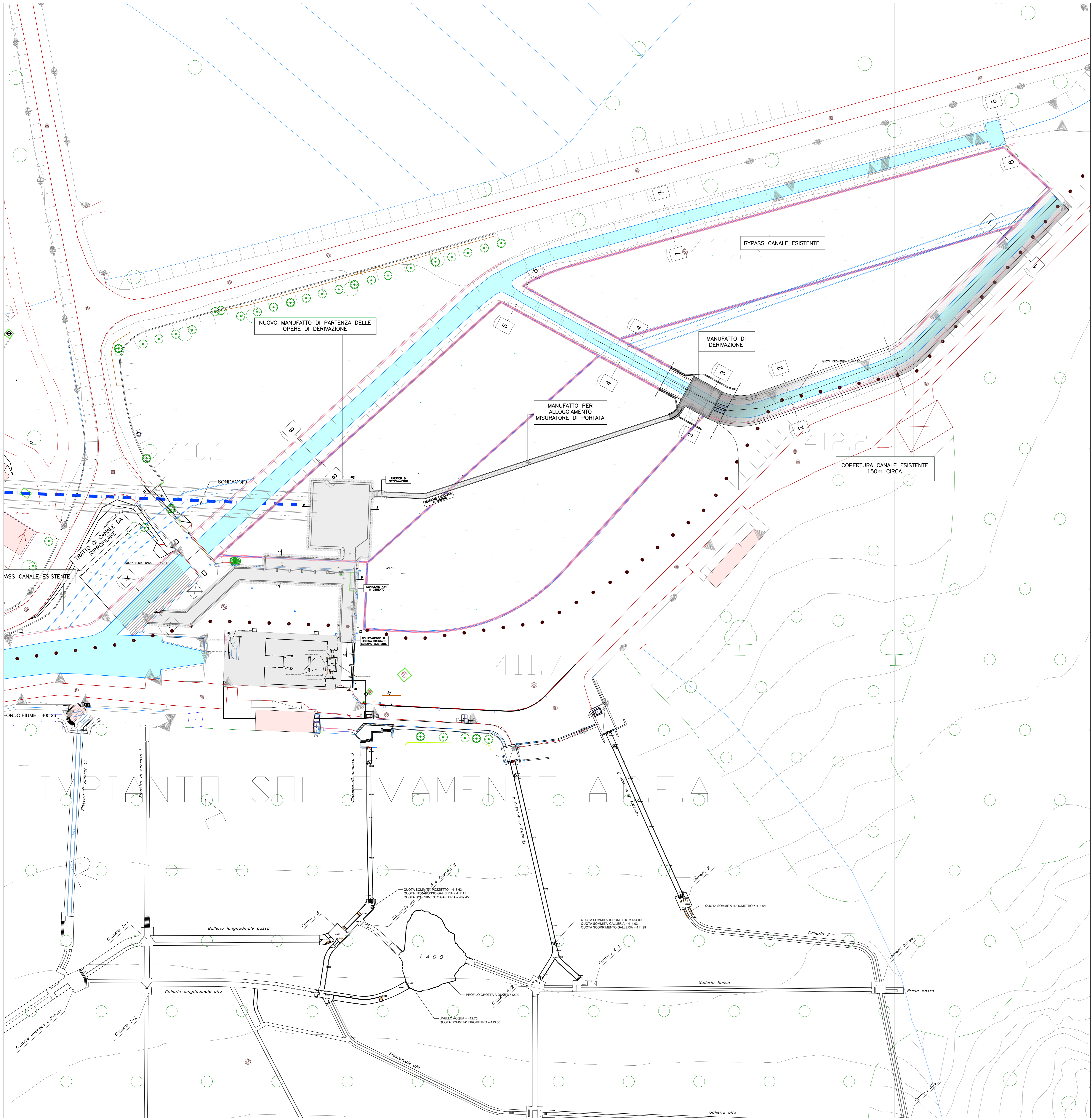
STRALCIO PLANIMETRICO - SCALA 1:500
