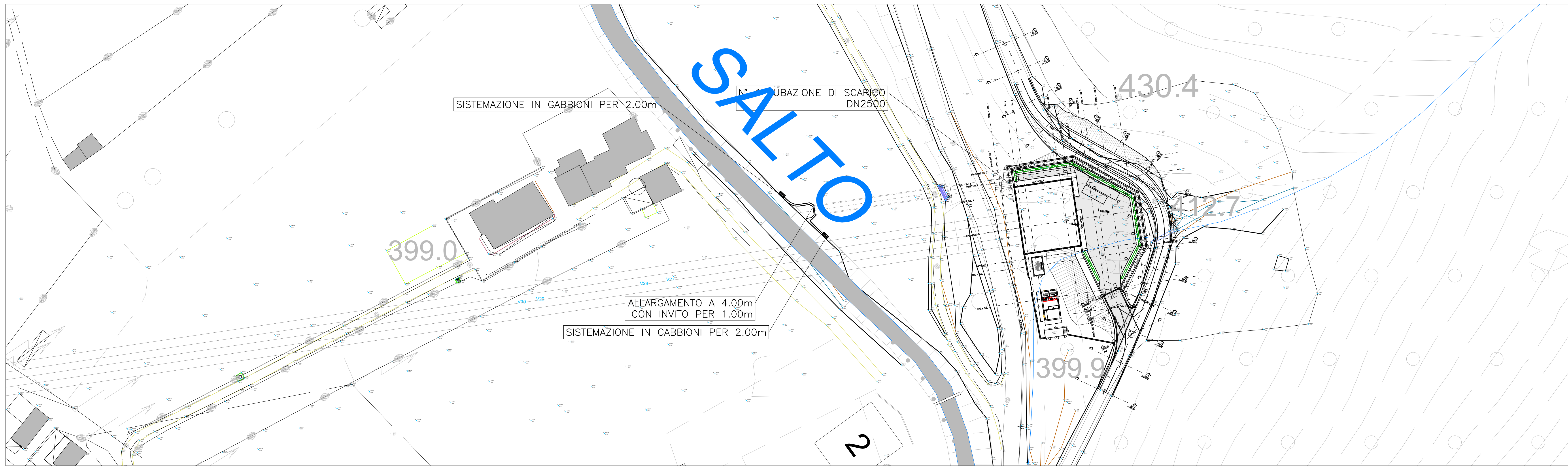
PLANIMETRIA GENERALE - Scala 1:1000
