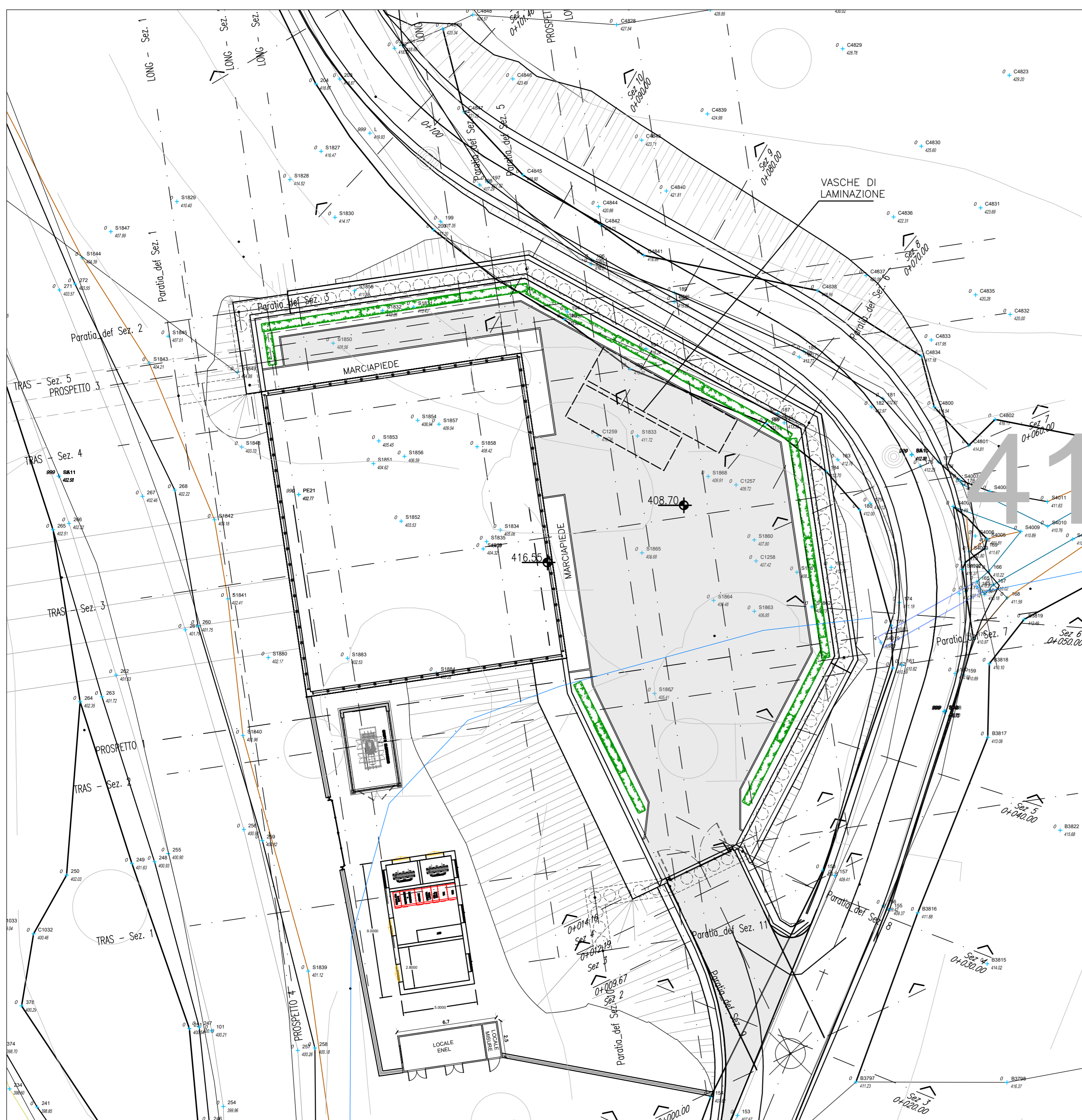
PLANIMETRIA GENERALE - Scala 1:500
