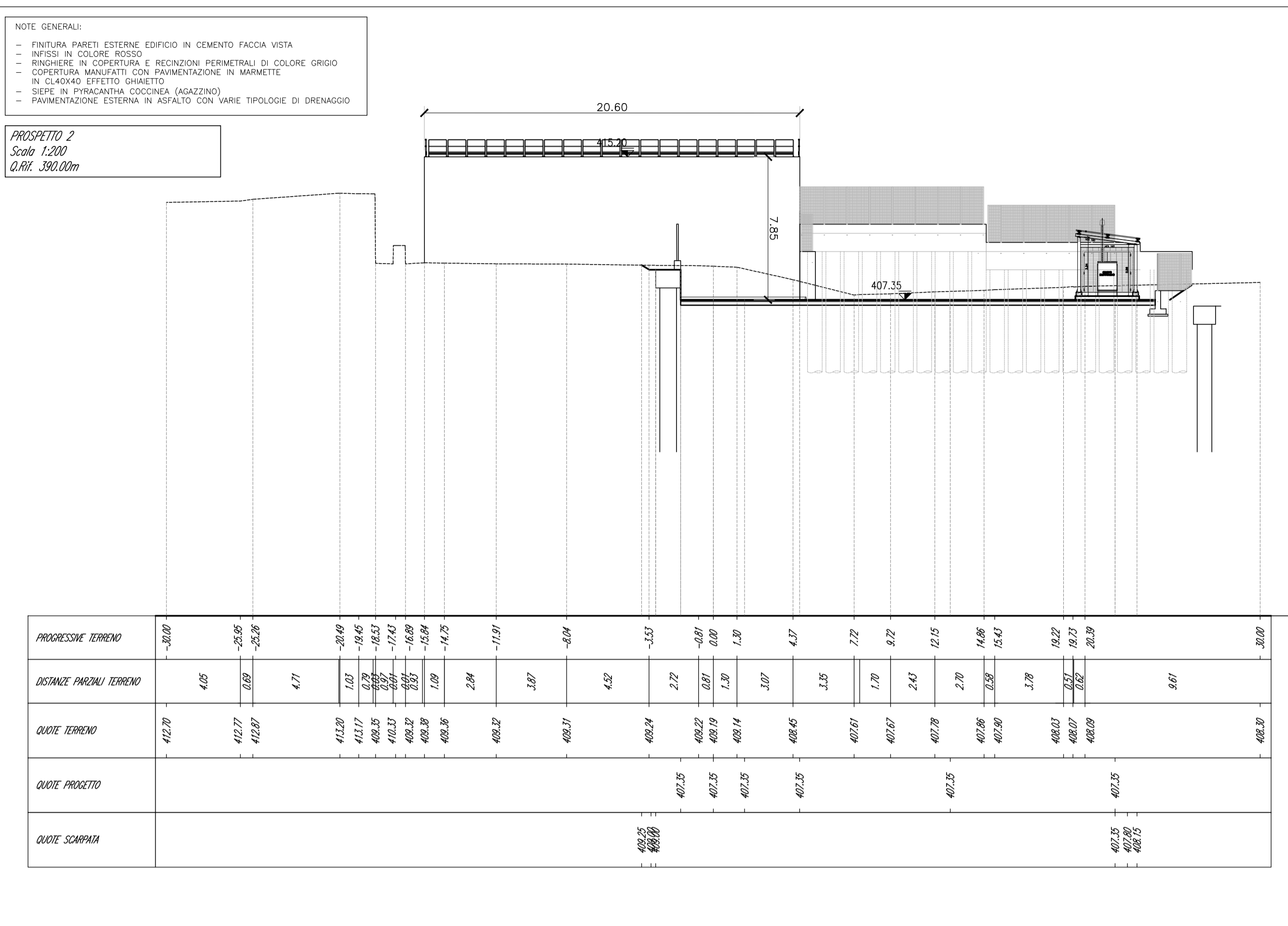
PROSPETTO 2 - SCALA 1:200
