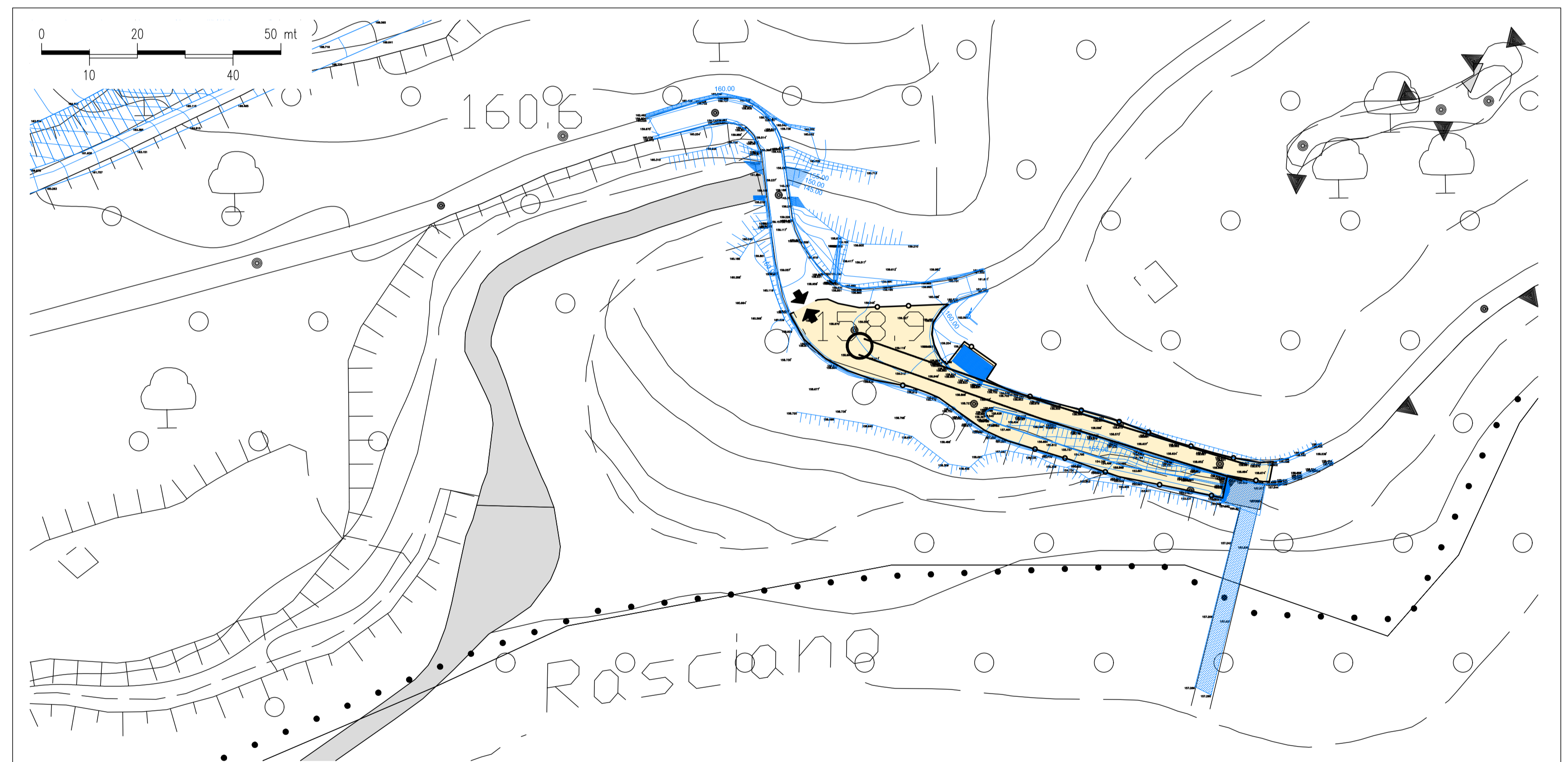
STRALCIO PLANIMETRICO COLLEGAMENTO AL TRONCO INFERIORE SX - SCALA 1:500
