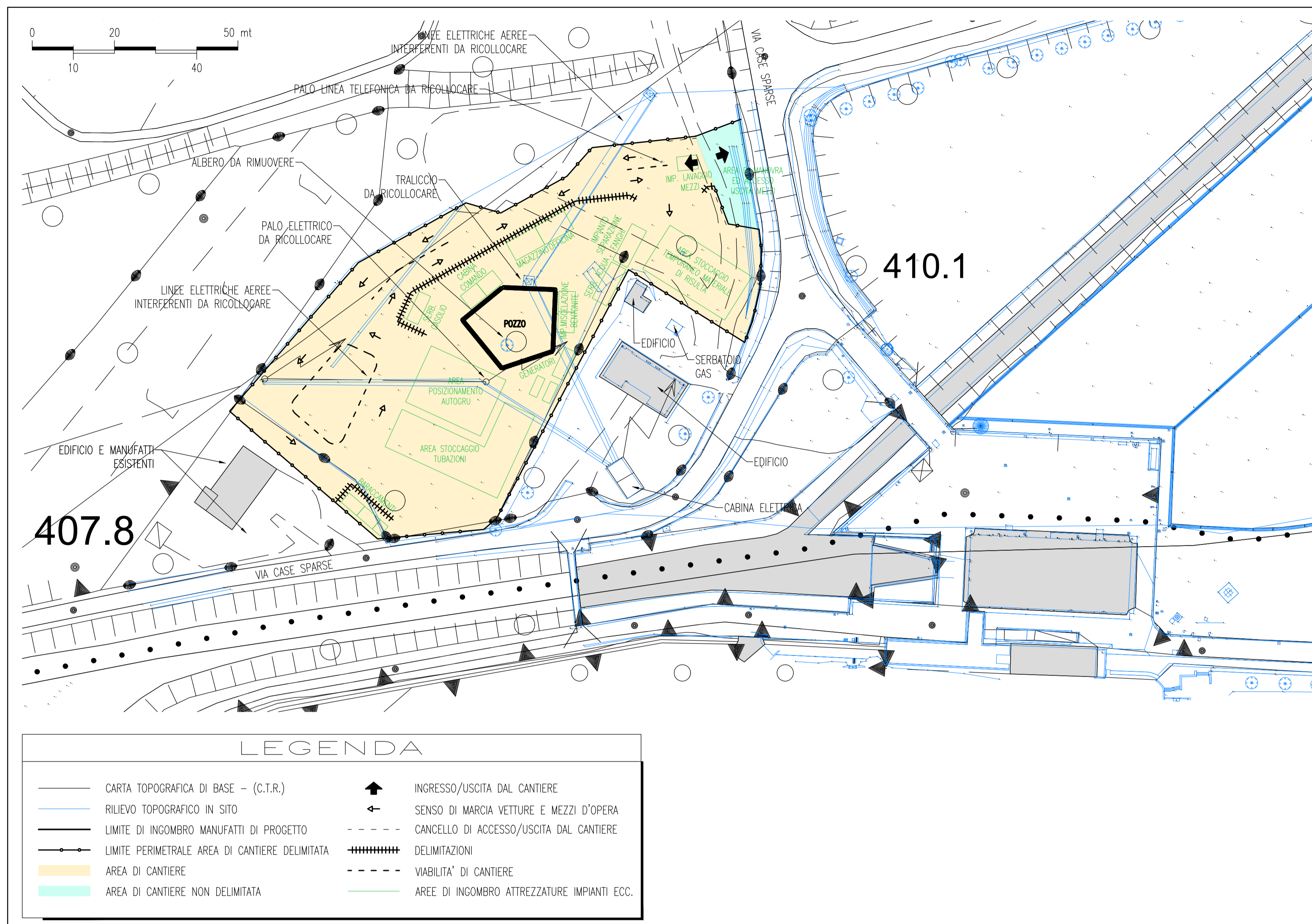
PLANIMETRIA DI CANTIERE
