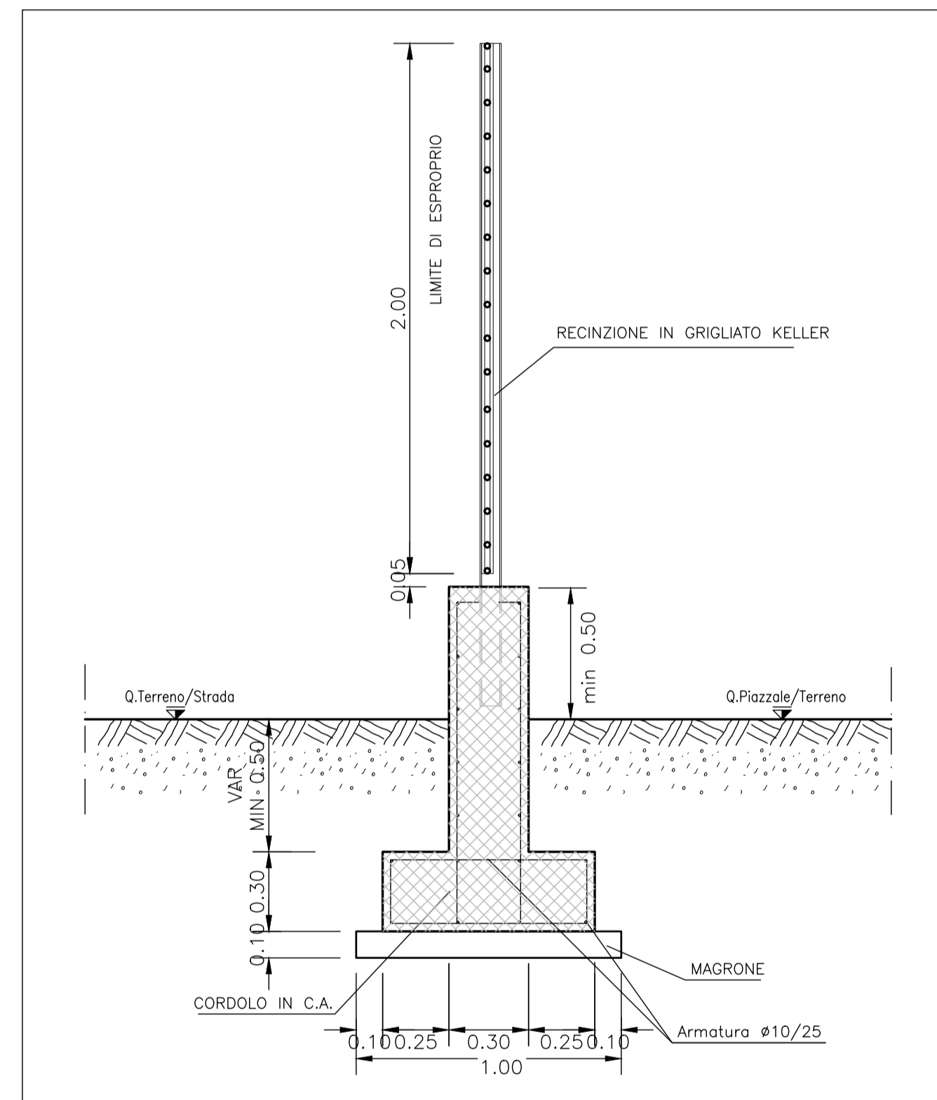
SEZIONE TIPO RECINZIONE - SCALA 1:200
