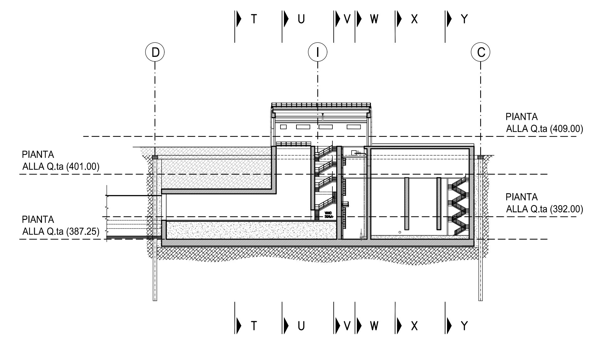
SEZIONE CHIAVE
