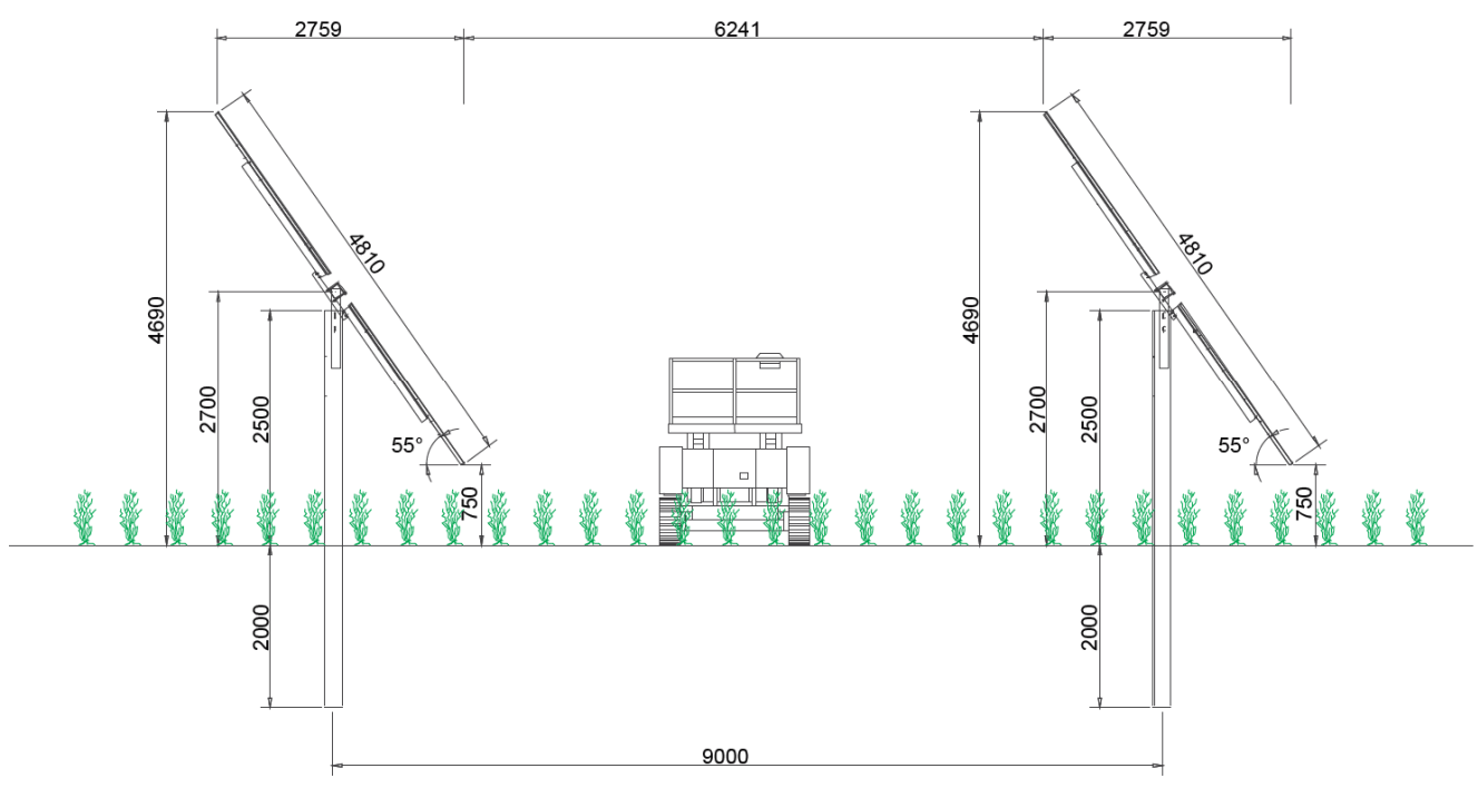
Figura 13 - Struttura di supporto con distanza tra i tracker e coltivazione sottostante
