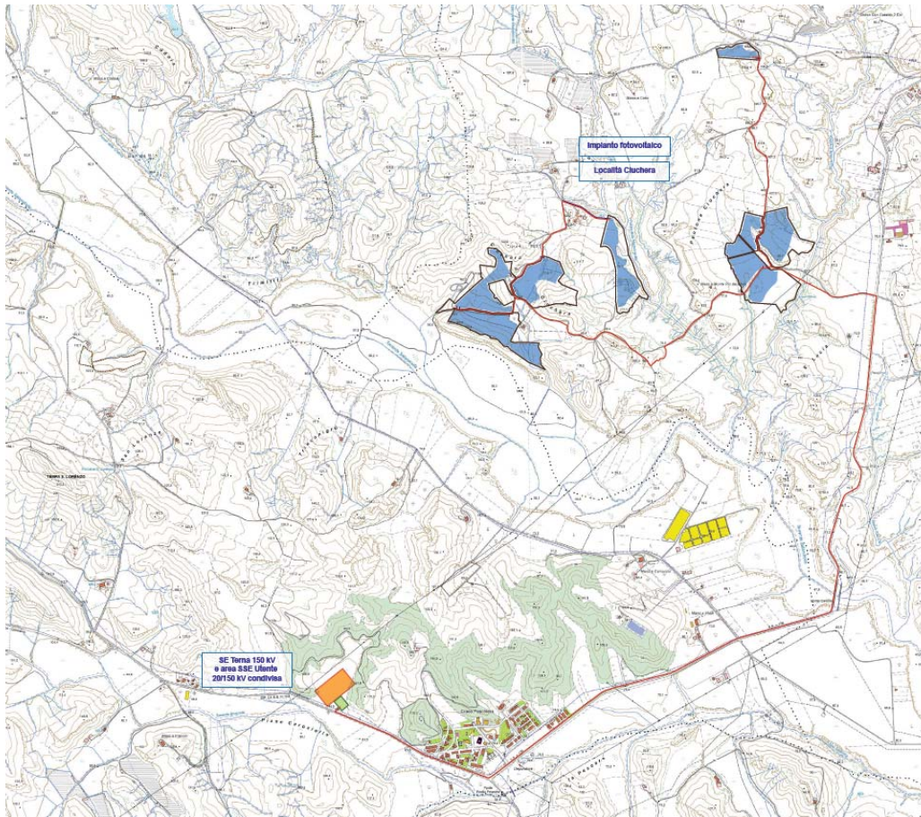
Figura 1 – Inquadramento dell'area di progetto su base CTR.
