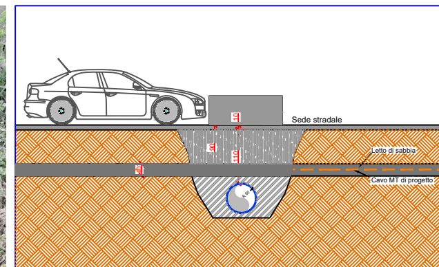
SEZIONE LONGITUDINALE 1:10
