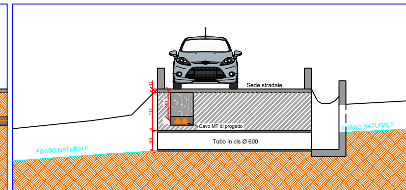
SEZIONE TRASVERSALE 1:10
