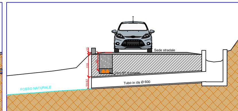
SEZIONE TRASVERSALE 1:10
