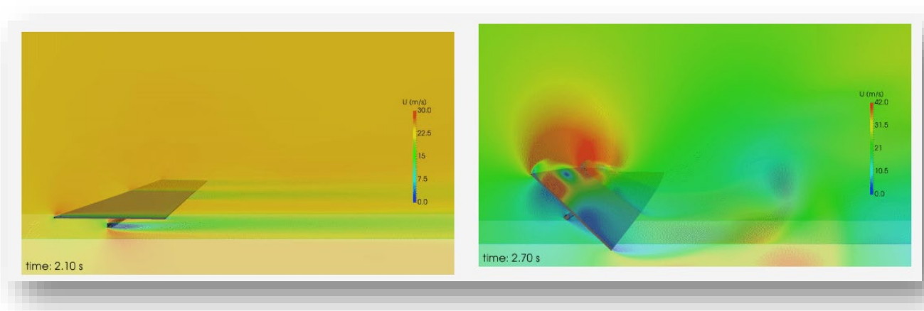
Figura 2 Simulazioni CFD eseguite da Soltec in collaborazione con Lynx basate sulla metodologia Dy-Wind
