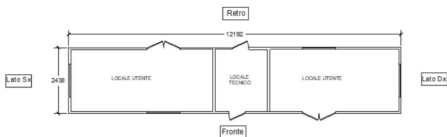
Planimetria cabina utente
