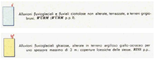
Stralcio carta geologica d'Italia scala 1:100.000
