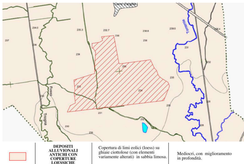
Stralcio Tav. G6 - Carta litotecnica del PRGC Masserano
