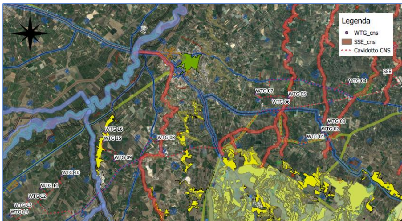
Figura 4 - Ipotesi di layout a 16 aerogeneratori - analisi vincolistica
