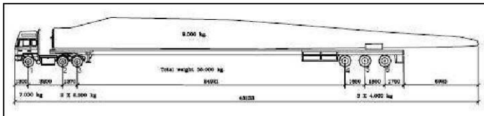
Figura 13 - Dimensioni autoarticolato
