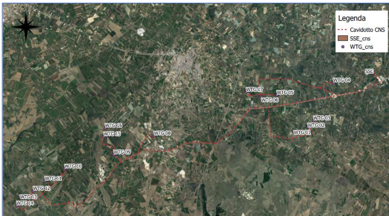
Figura 3 - Ipotesi di layout a 16 aerogeneratori
