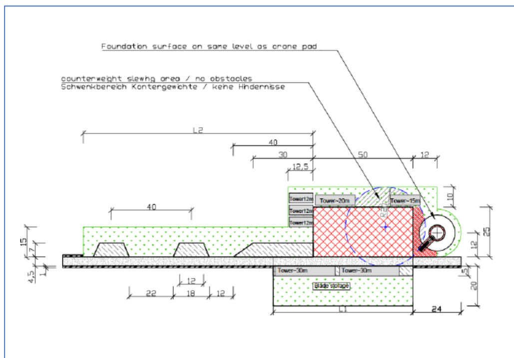
Figura 16 – tipologico della piazzola di montaggio
