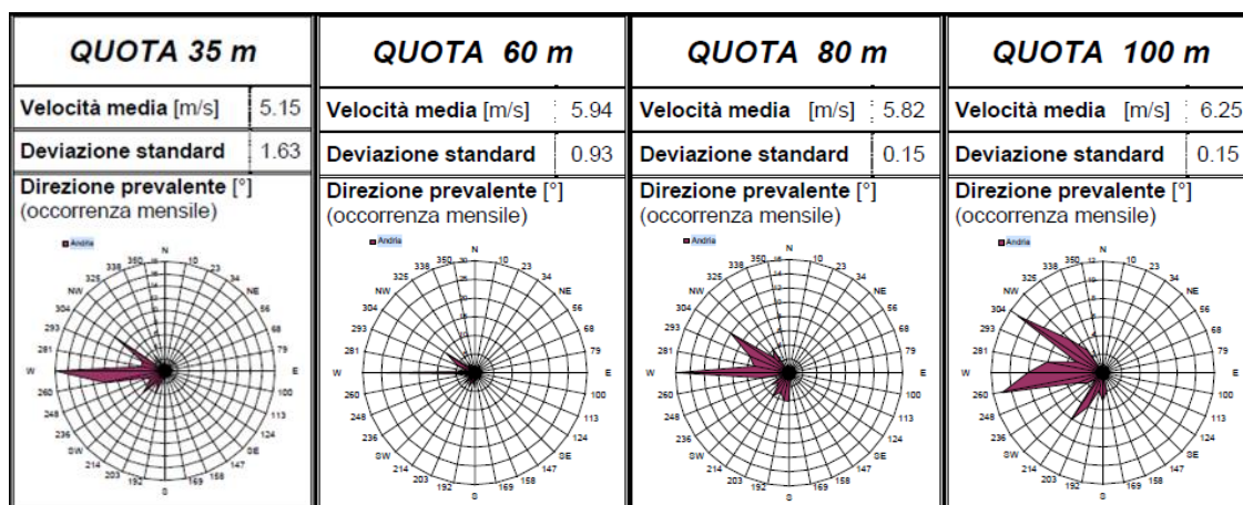
Andria – Atlante eolico della Puglia
