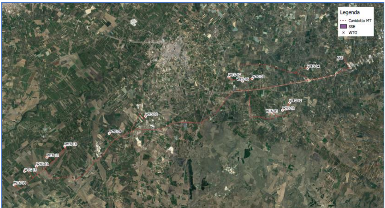
Figura 6 - layout impianto definitivo a n.14 aerogeneratori
