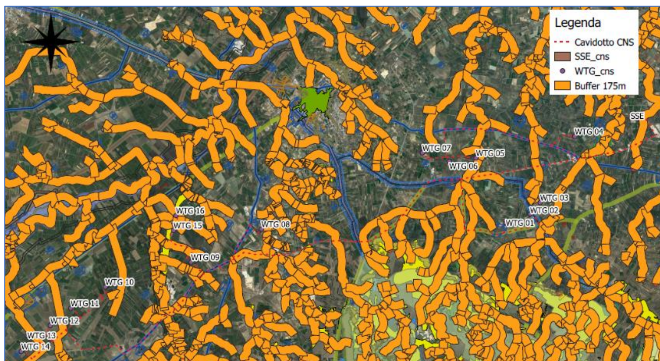
Figura 5 - Ipotesi di layout a 16 aerogeneratori - analisi vincolistica e buffer dai canali
