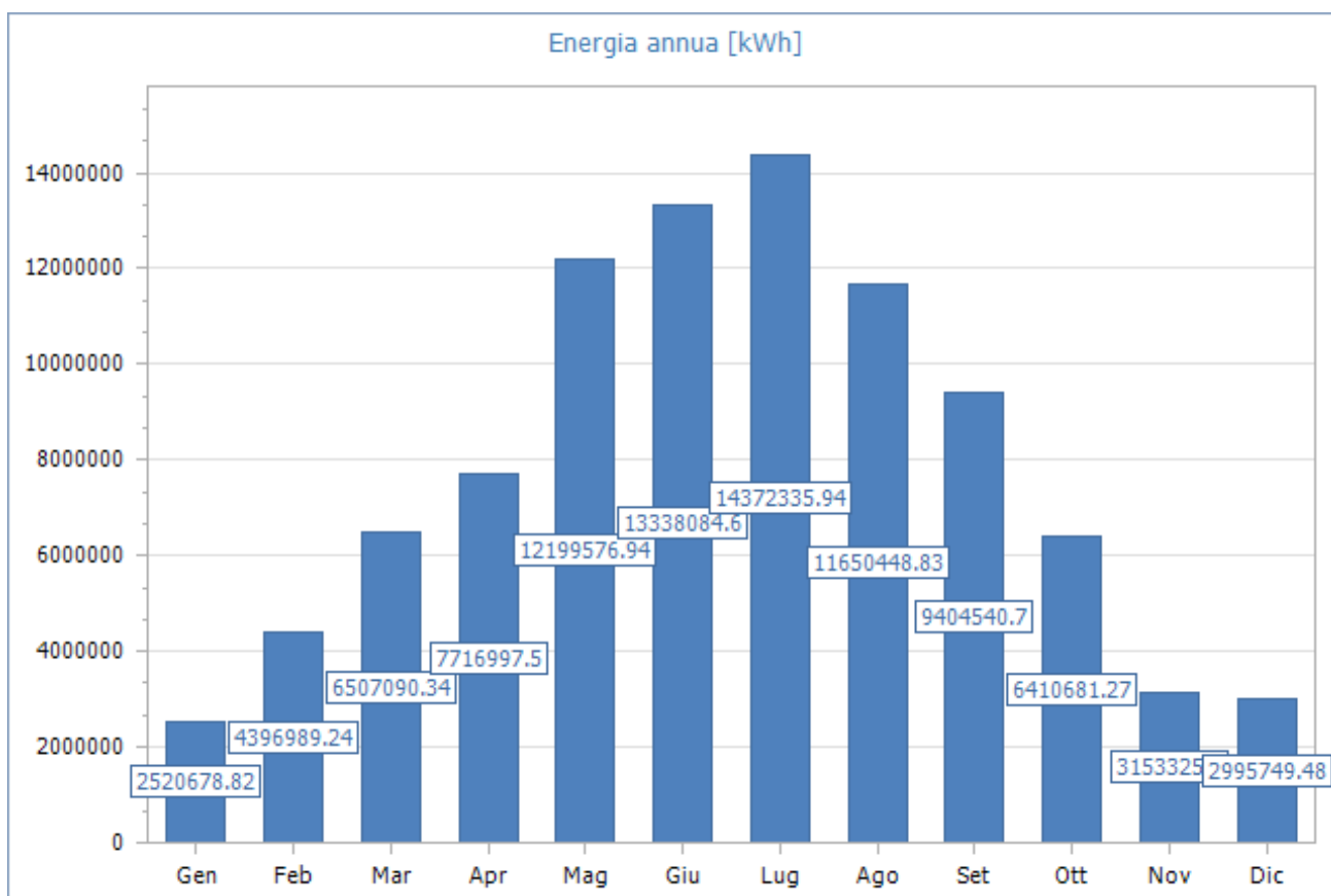
Fig. 2: Energia mensile prodotta dall'impianto
