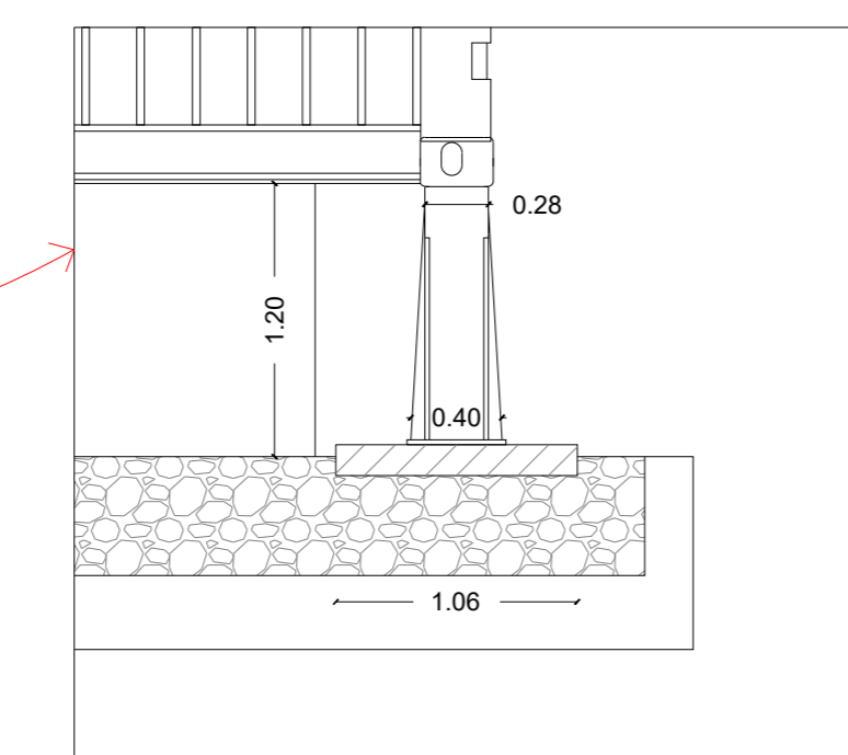
PARTICOLARE PIEDE D'APPoggio
