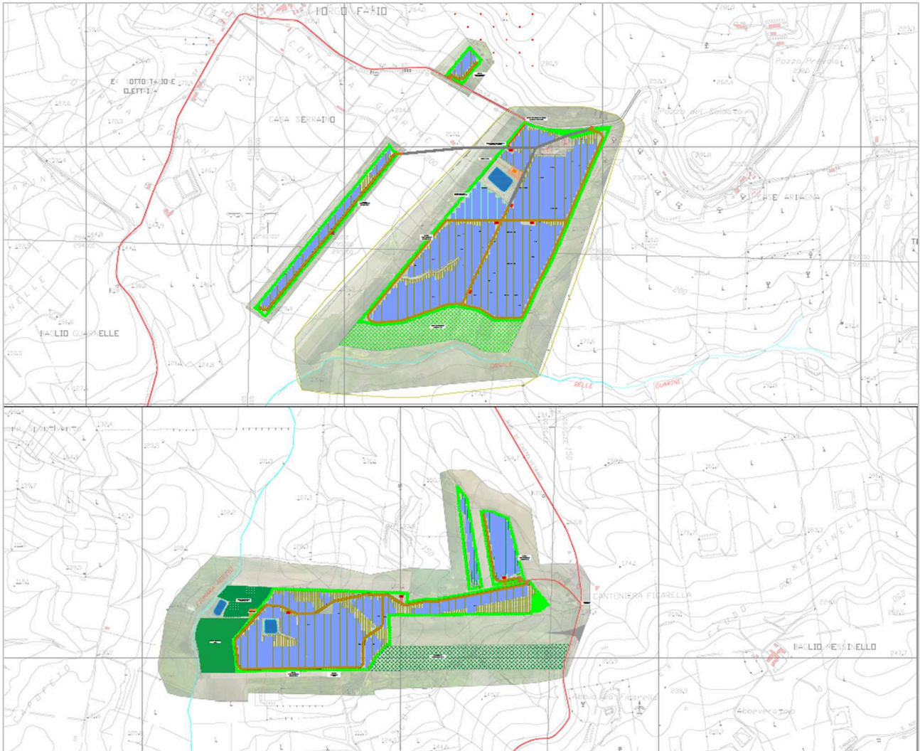
Lay-out generale dell'impianto agrovoltaico (Elaborato XE-CUDDIA-AFV-PD-D-1.6.0.0)
