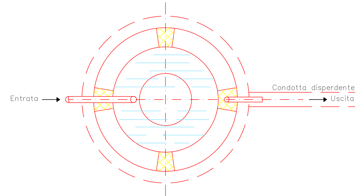
FOSSA IMHOFF - PARTICOLARE COSTRUTTIVO SCALA 1:10
