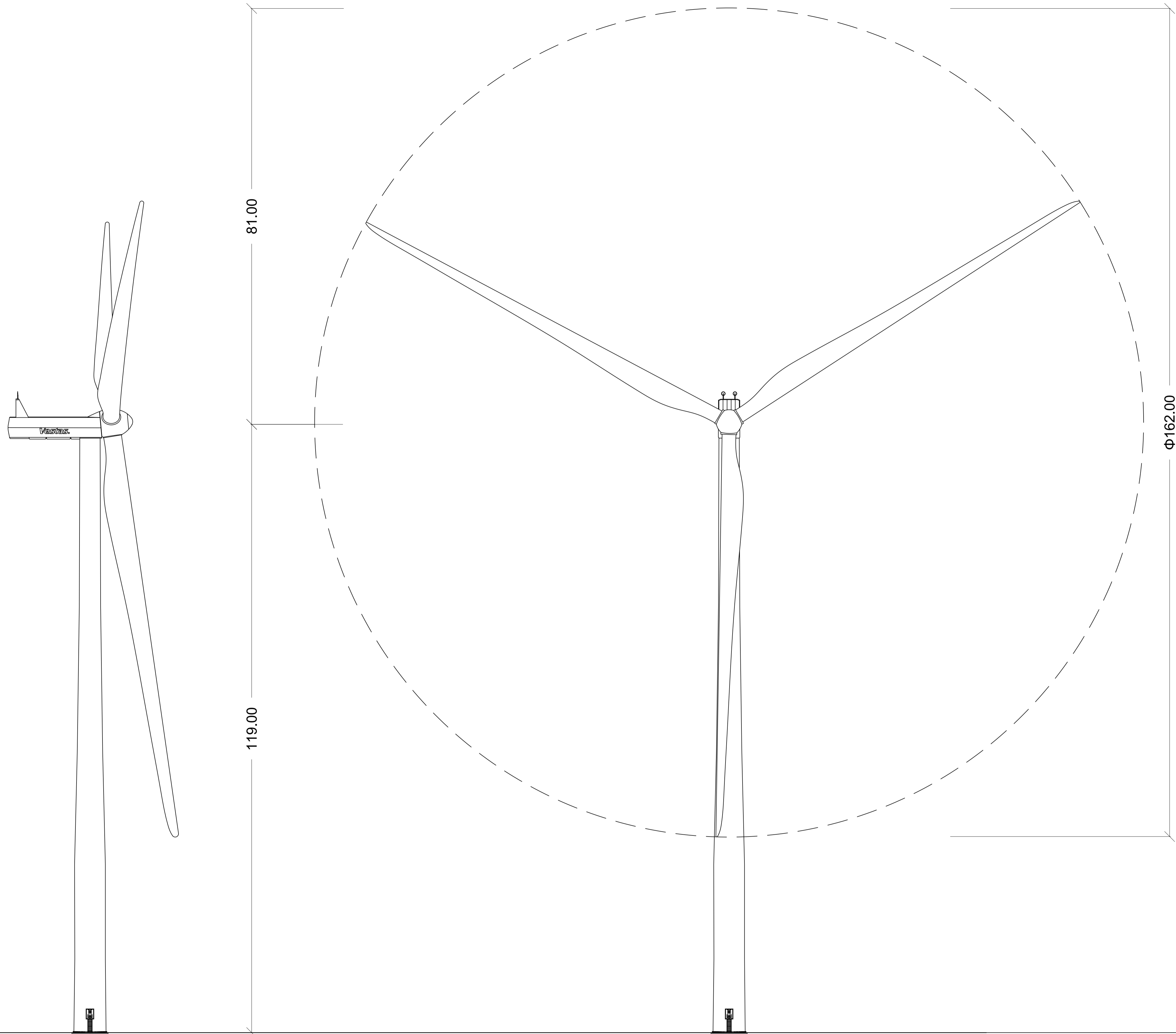
VISTA FRONTALE - SCALA 1:400
