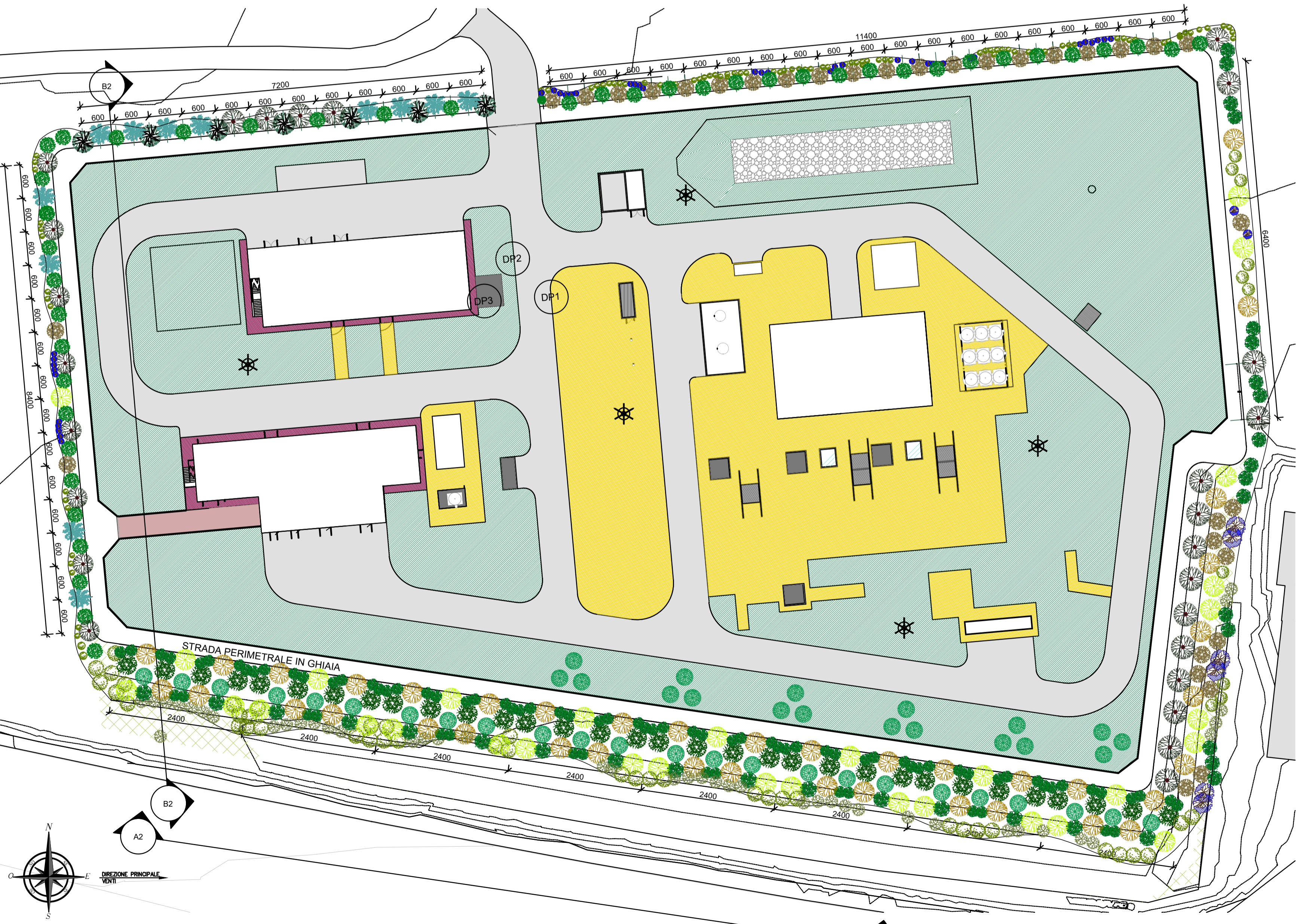
PLANIMETRIA - SESTI DI IMPIANTO Scala 1: 500
