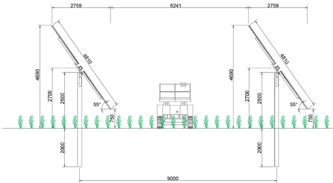
Figura 15 - Struttura di supporto con distanza tra i tracker.
