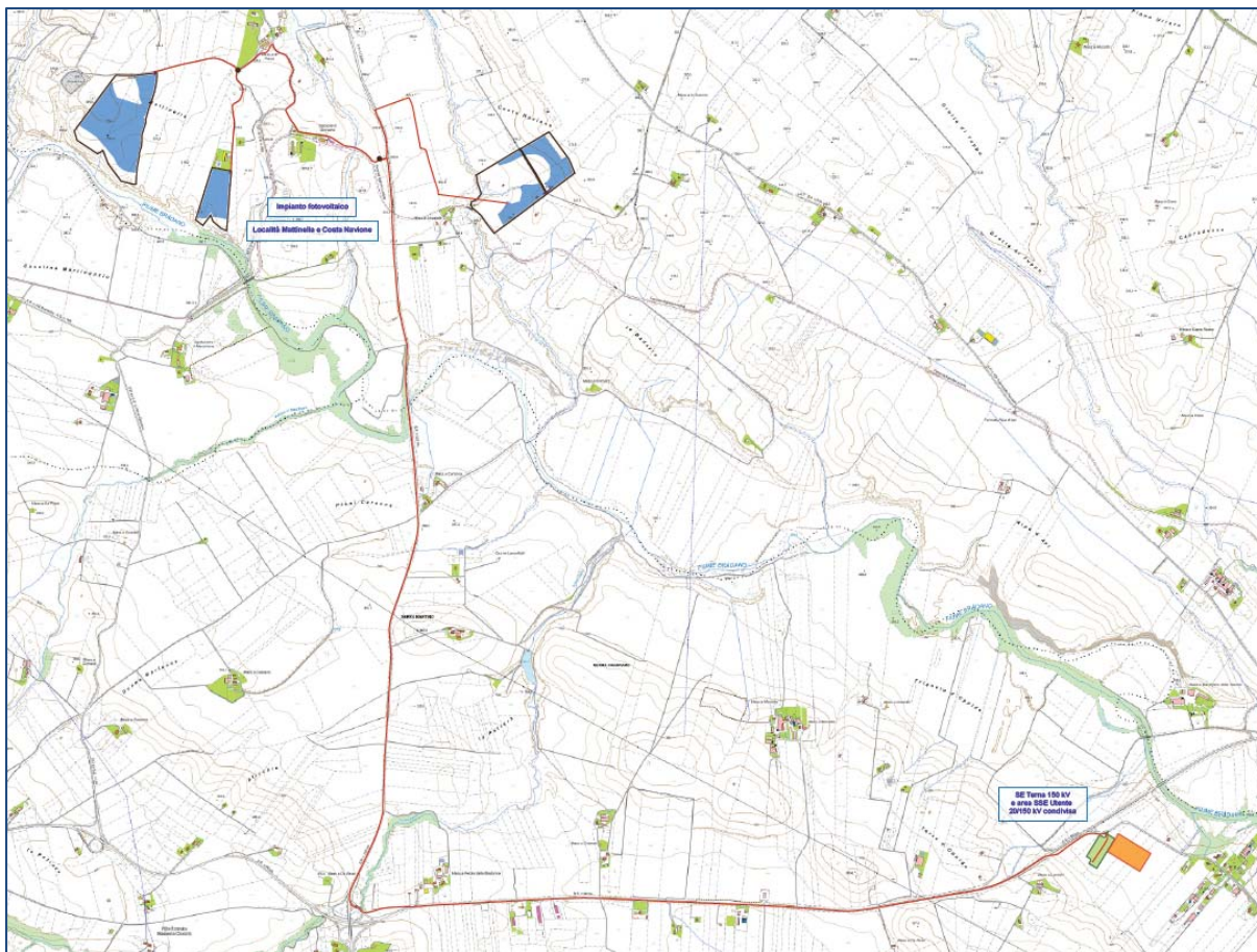
Figura 1 – Inquadramento dell’area di progetto su base CTR.
