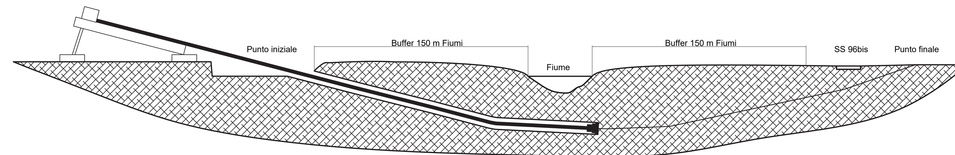
Interferenza cavidotto / Corso d'acqua TRIVELLAZIONE ORIZZONTALE CONTROLLATA (TOC)
