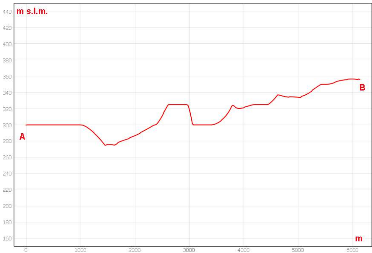
Sezione morfologica del terreno- Punto di presa n°11
