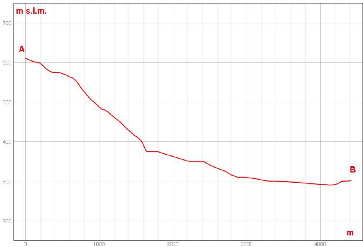
Sezione morfologica del terreno- Punto di presa n°8
