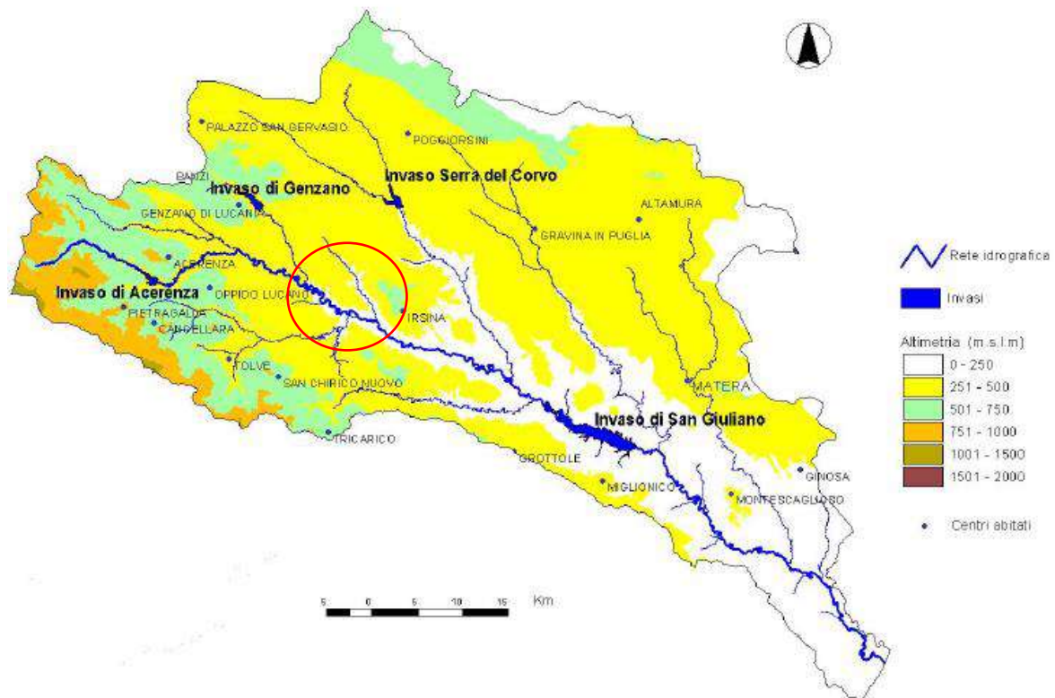
Figura 5.15. – Bacino Idrografico del fiume Bradano.
