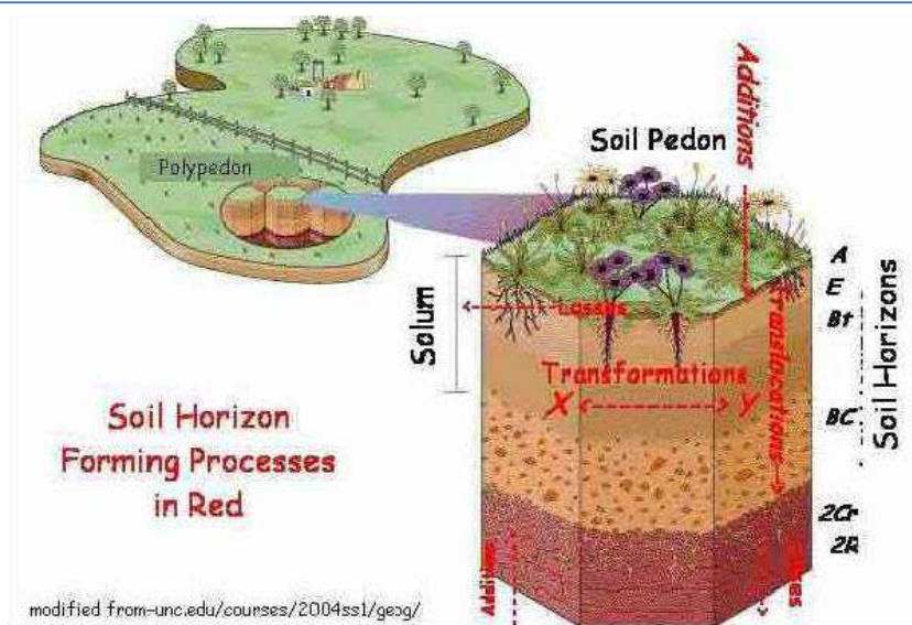
Figura 8.21. – Unità rappresentativa del suolo – PEDON.
