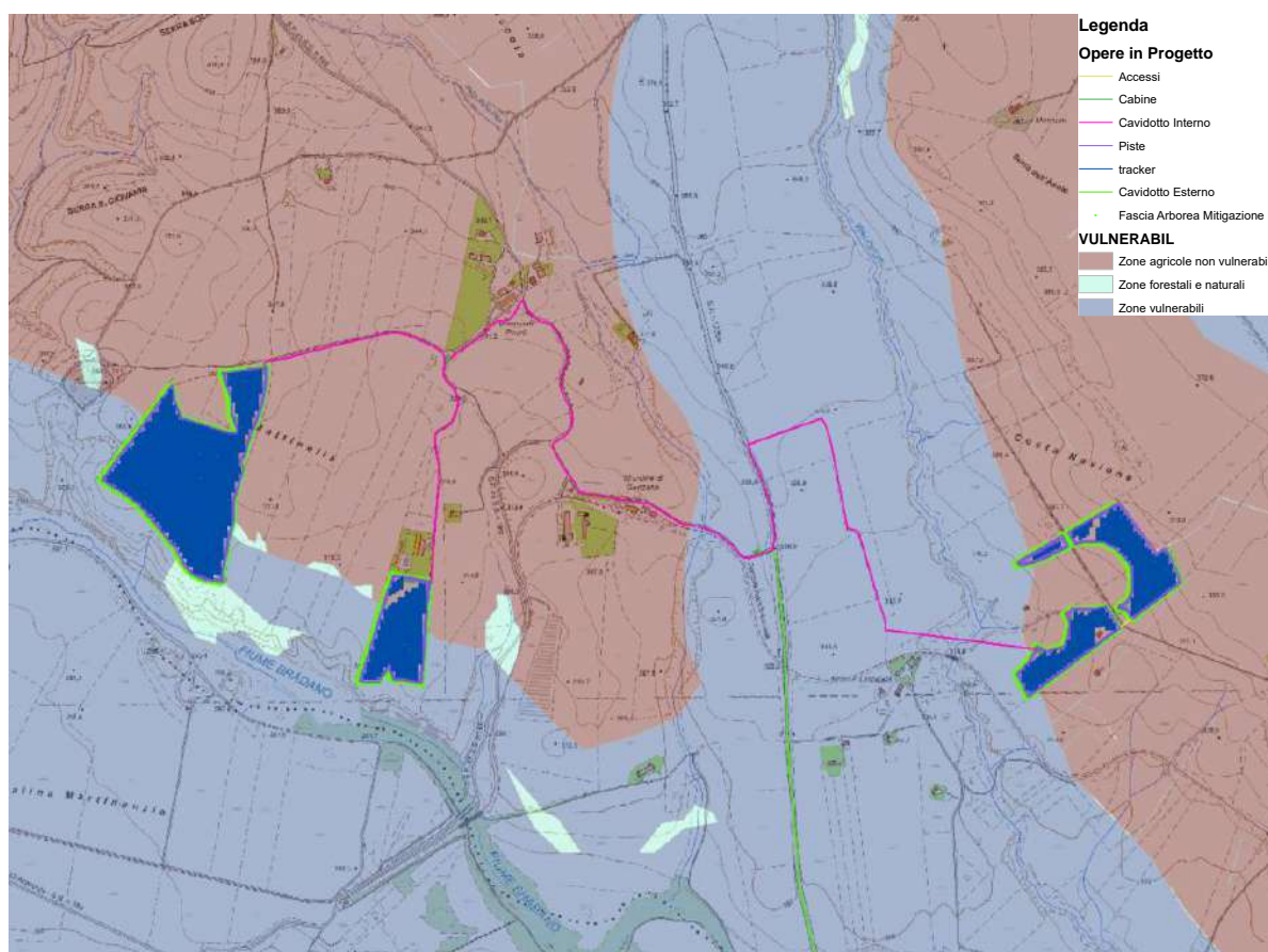
Figura 8.23 – Carta della Vulnerabilità da nitrati di origine agricola.
