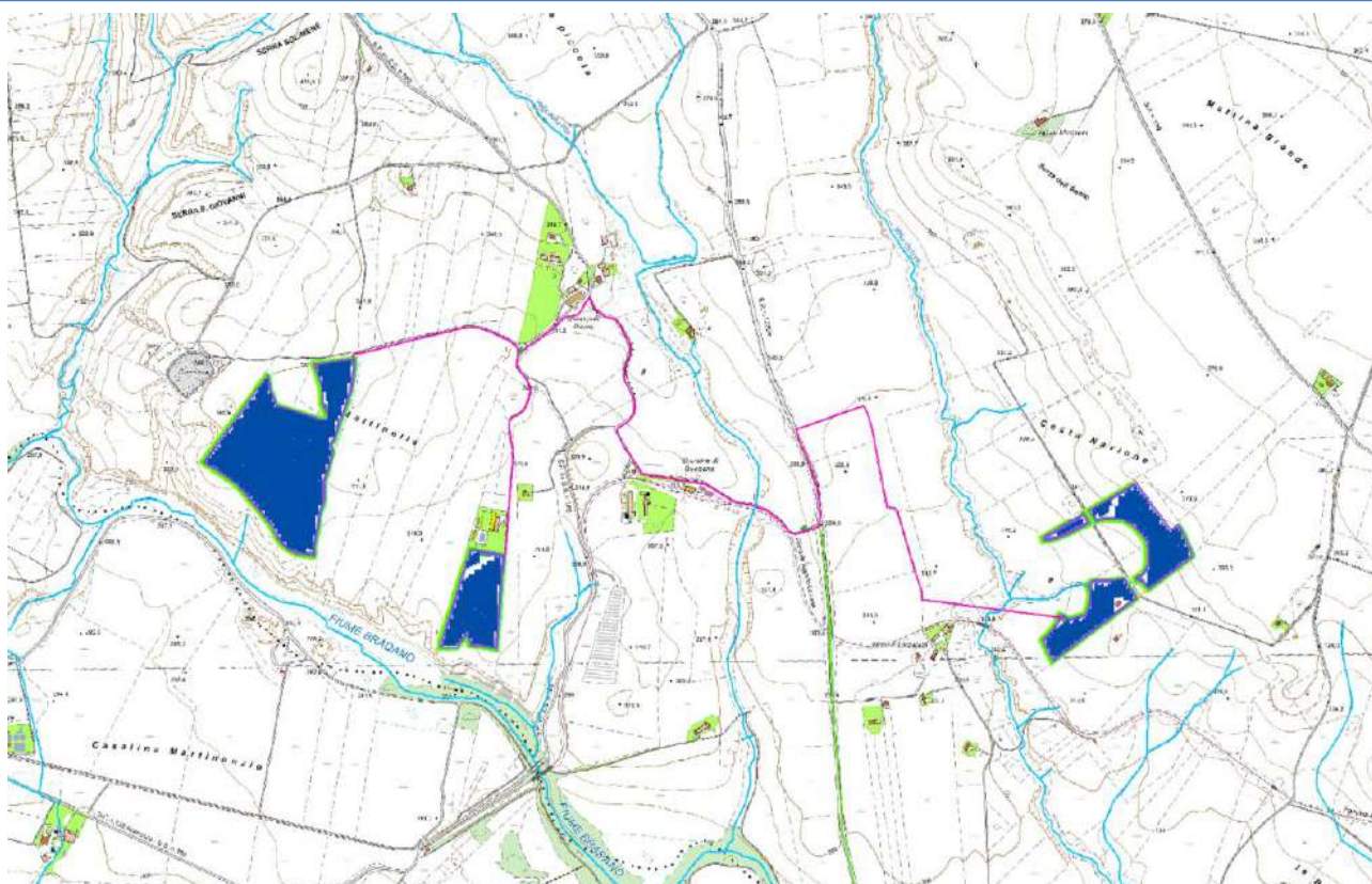
Figura 8.20. – Dettaglio dell'Idrografia dell'area su CTR
