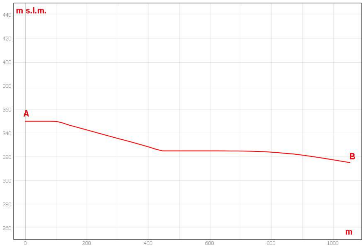
Figura 11.12. – Sezione morfologica del terreno- Punto di presa n°2
