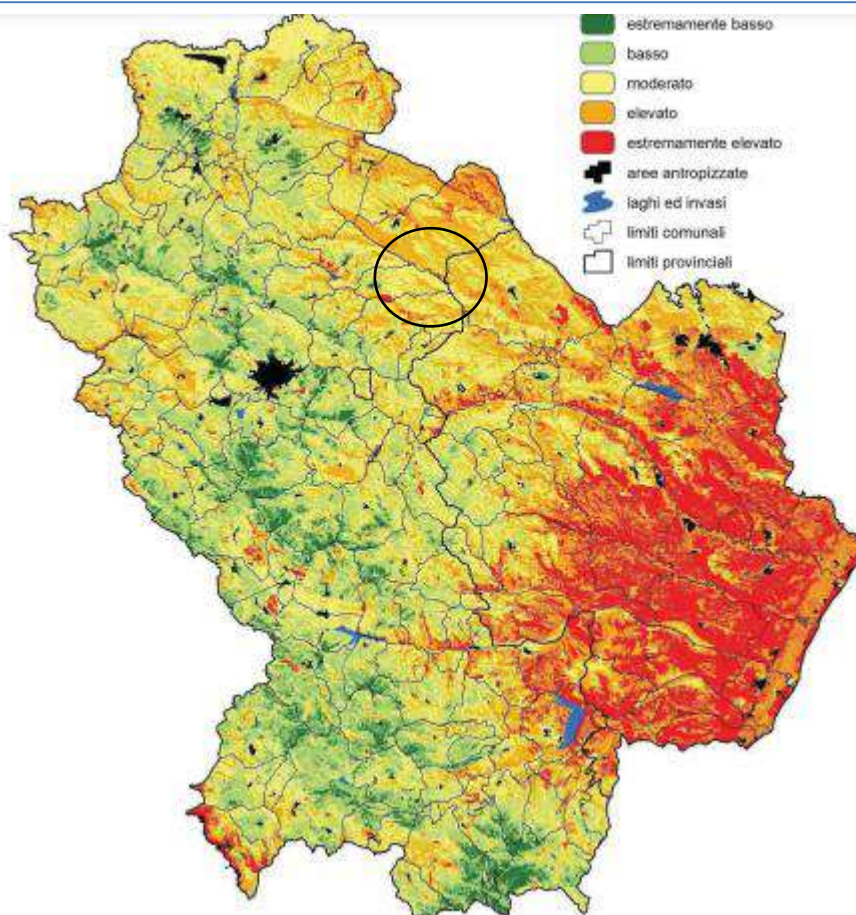
Figura 5.21. – Carta del rischio incendio della Regione Basilicata (CRDI)
