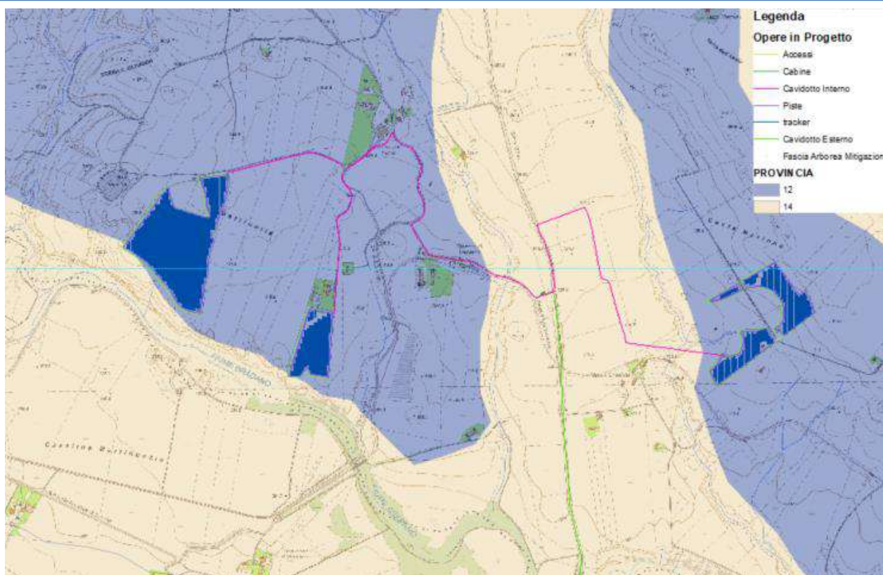
Figura 8.26. – Province Pedologiche area di progetto.
