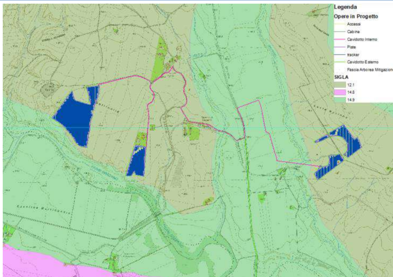
Figura 8.27. – Unità Pedologiche area di progetto.
