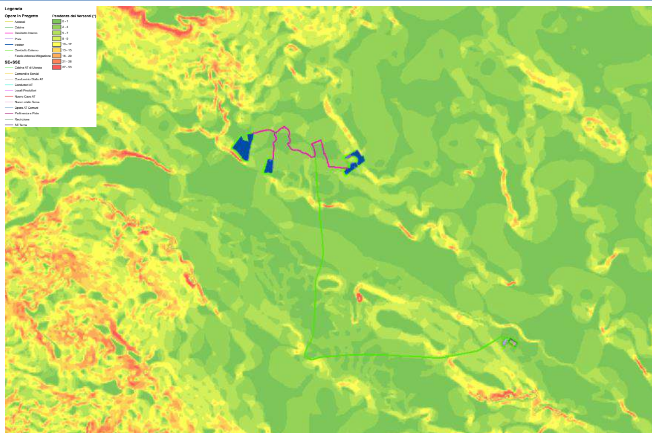
Figura 8.15. – Stralciamento Carta delle pendenze area di progetto.
