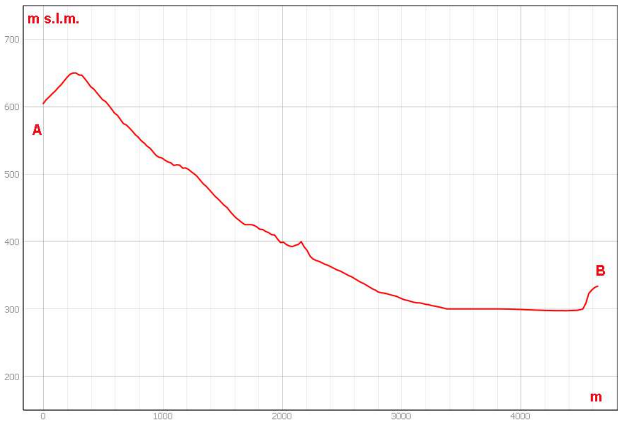
Sezione morfologica del terreno- Punto di presa n°7
