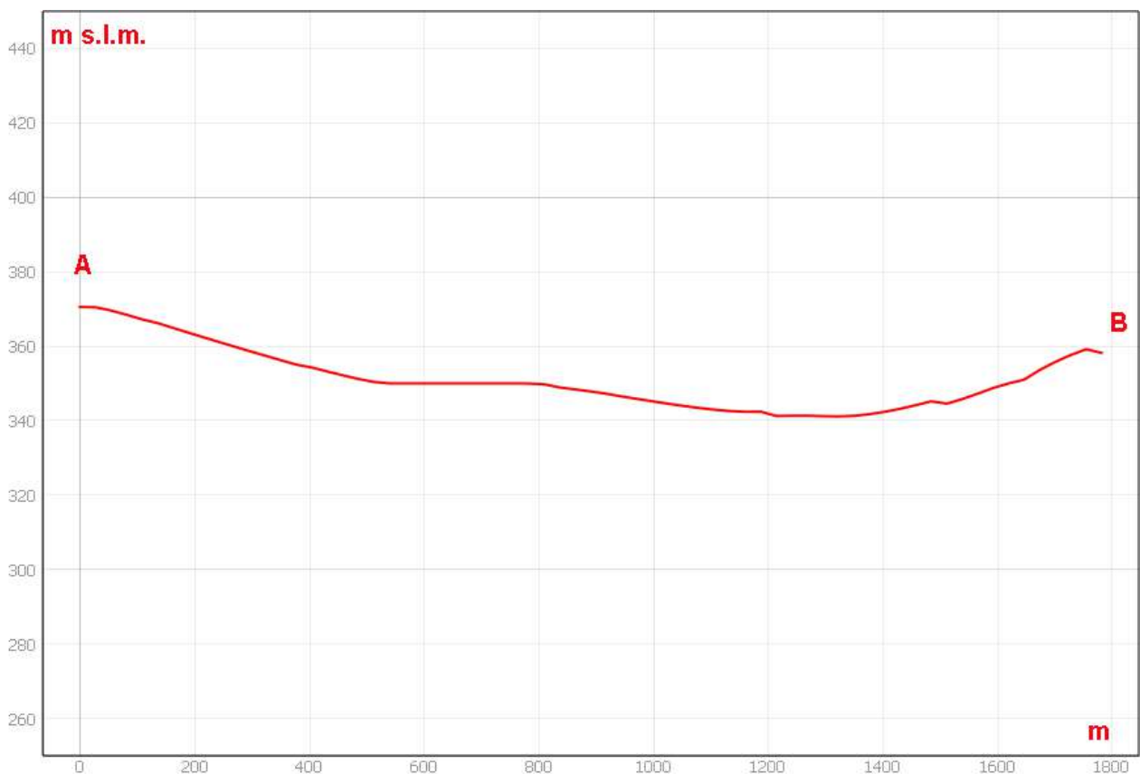
Figura 11.8. – Sezione morfologica del terreno- Punto di presa n°1
