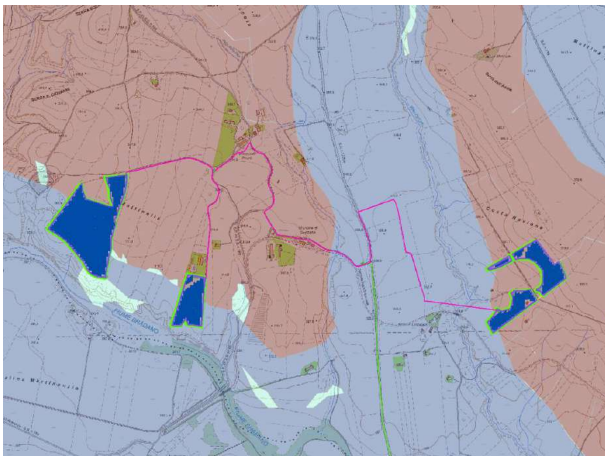
Figura 13.1. – Carta della Vulnerabilità da nitrati di origine agricola.
