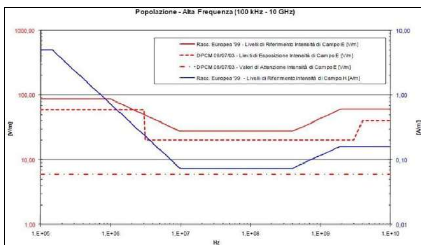
Figura 13.8. – Livelli esposizione Alta Frequenza (100Hz – 10 GHz).
