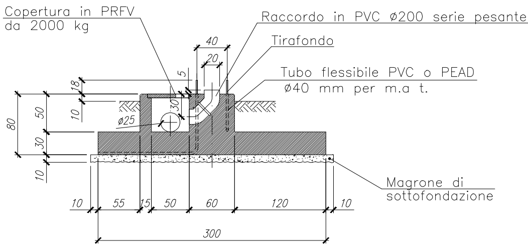
SEZIONE 2-2
