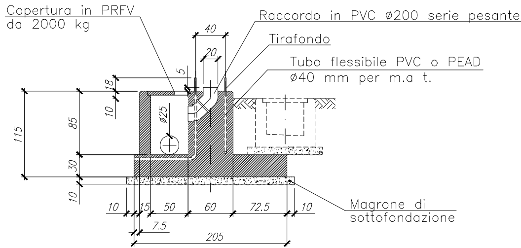
SEZIONE 1-1
