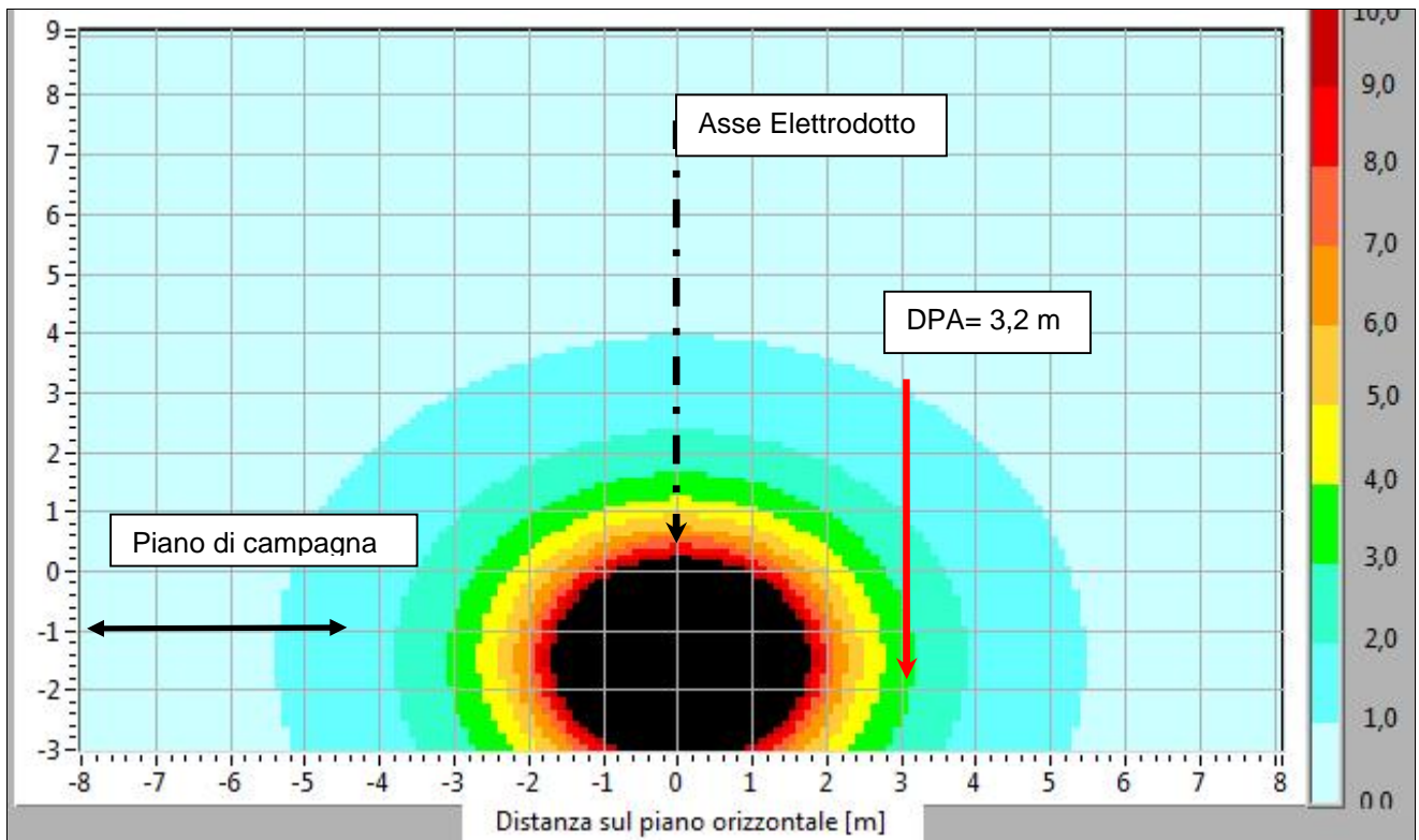
Fig. 4 Mappa verticale induzione magnetica (B) sezione tipo con indicazione della DPA - V=150 kV I = 1045 A
