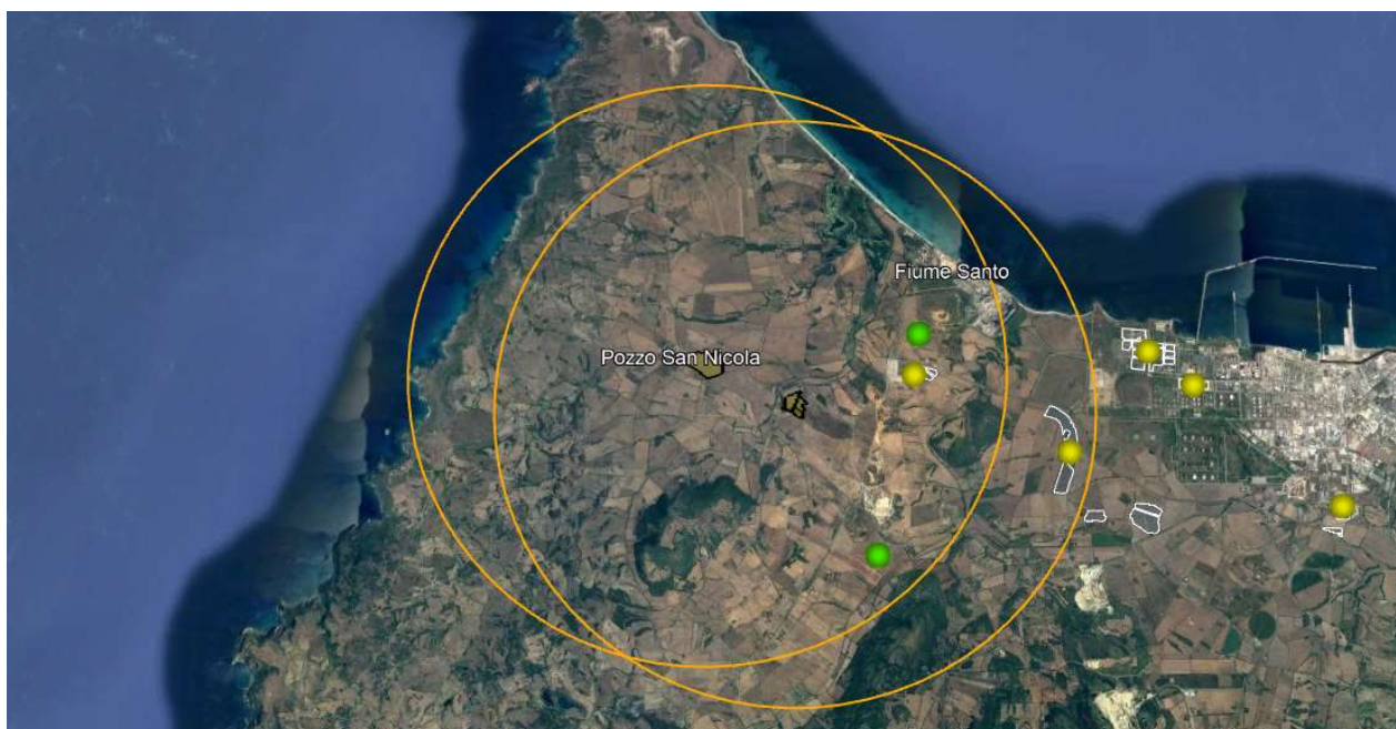
FIGURA 49 – IMPIANTI FV (IN ●) E IMPIANTI EOLICI (IN ●) PRESENTI NEL RAGGIO DI 5 KM (IN ARANCIO) DALLE AREE DI PROGETTO (IN GIALLO)
