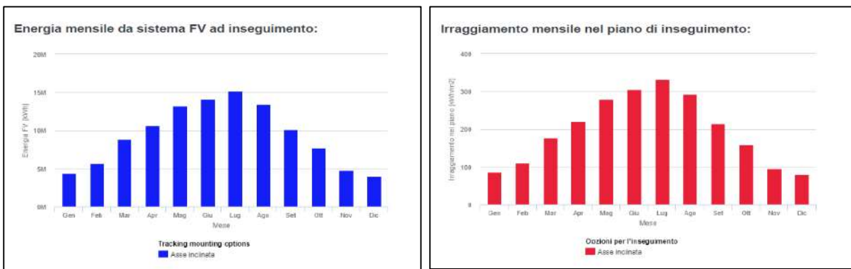
FIGURA 20 – SULLA SINISTRA PRODUCIBILITÀ MEDIA MENSILE DEL SITO, SULLA DESTRA IRRAGGIAMENTO AL METRO QUADRO – INFORMAZIONE ESTRATTA DALLA RELAZIONE TECNICA DI DETTAGLIO E CALCOLI PRELIMINARI STINTINO-PDR02
