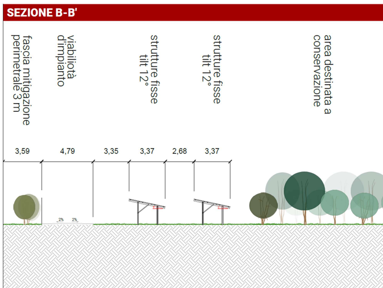
FIGURA 40 – SEZIONE N-S DELL'IMPIANTO – ESTRATTO DALL'ELABORATO GRAFICO STINTINO-PDT11)
