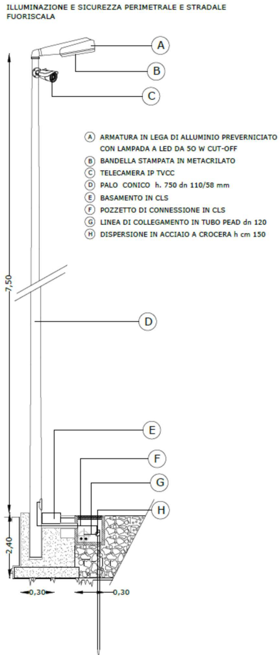
FIGURA 22 – ESEMPIO IMPIANTO DI ILLUMINAZIONE INTEGRATO CON SISTEMA DI VIDEOSORVEGLIANZA – ESTRATTO DALL'ELABORATO TECNICO STINTINO-PDR02
