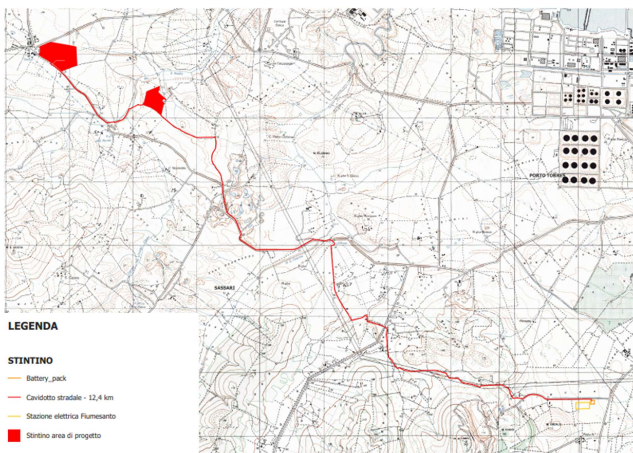
FIGURA 34 – ESTENSIONE AREA DI PROGETTO SU CARTOGRAFIA IGM IN SCALA 1:25.000. IN ROSSO I POLIGONI DELL'AREA DI PROGETTO E IL CAVIDOTTO – ESTRATTO DALL'ELABORATO CARTOGRAFICO STINTINO-IAT01
