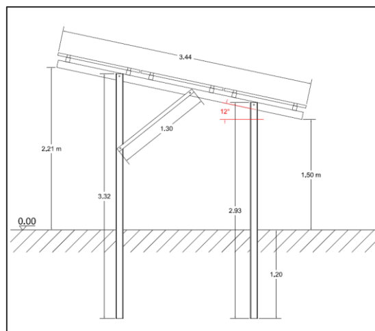
FIGURA 2: SCHEMA TIPO STRUTTURA FISSA PROPOSTA
