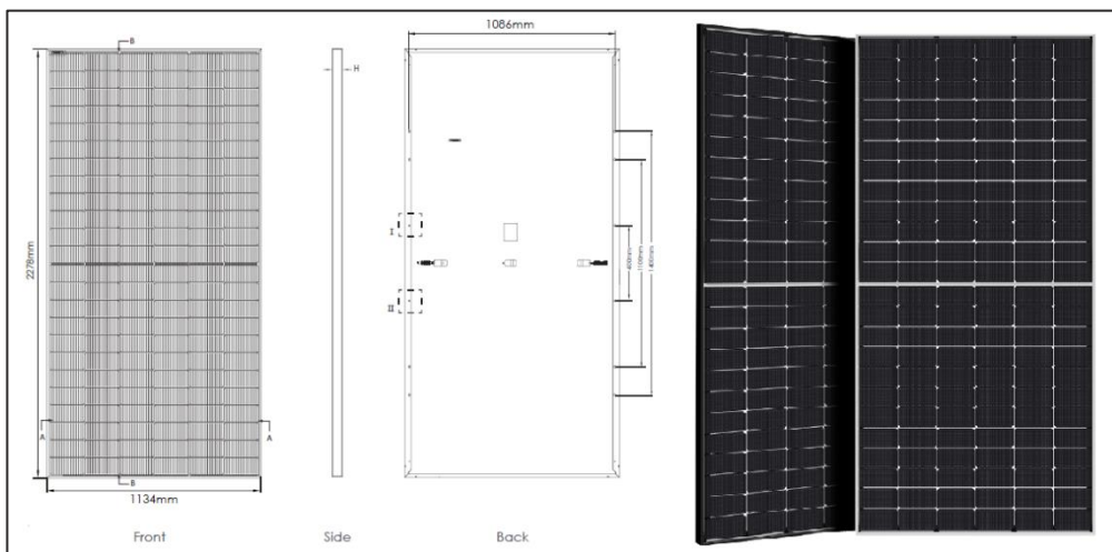
FIGURA 5: PANNELLO FV PARI A 570 WP CON DIMENSIONI 2278 × 1134 × 35 MM
