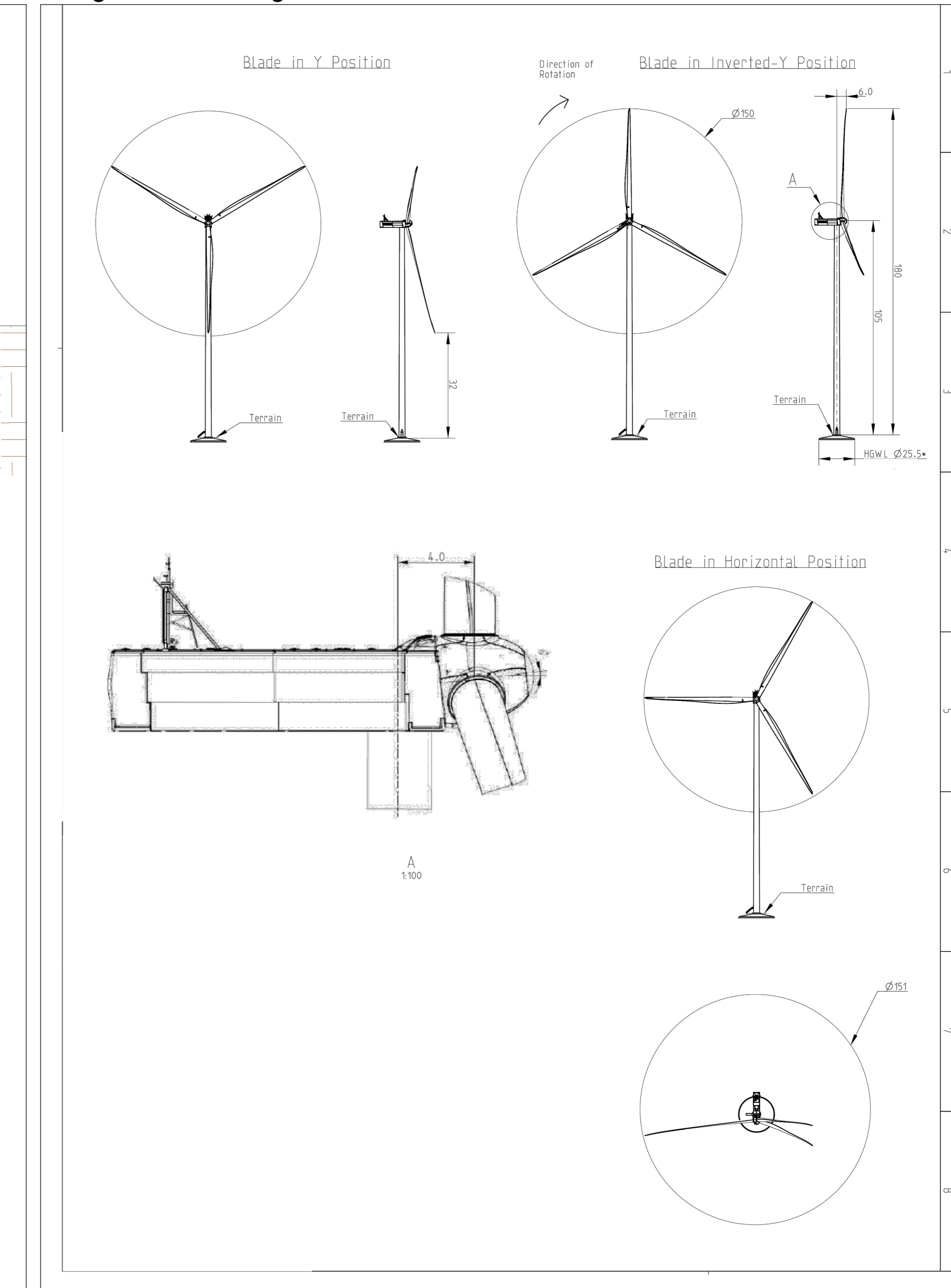
Disegni tecnici aerogeneratore
