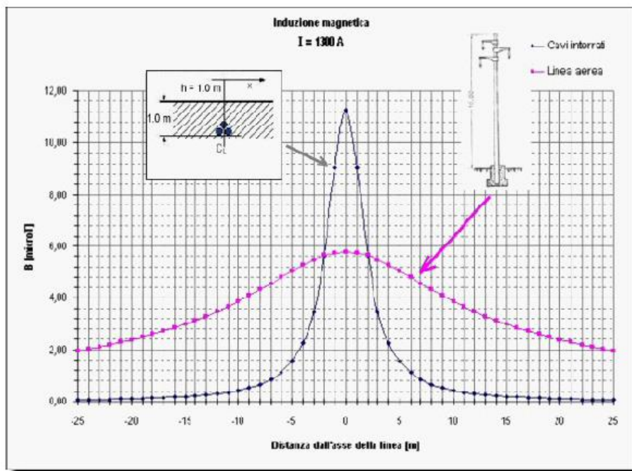
Figura 1: Attenuazione dell'induzione magnetica dovuta all'interrimento dei cavi
