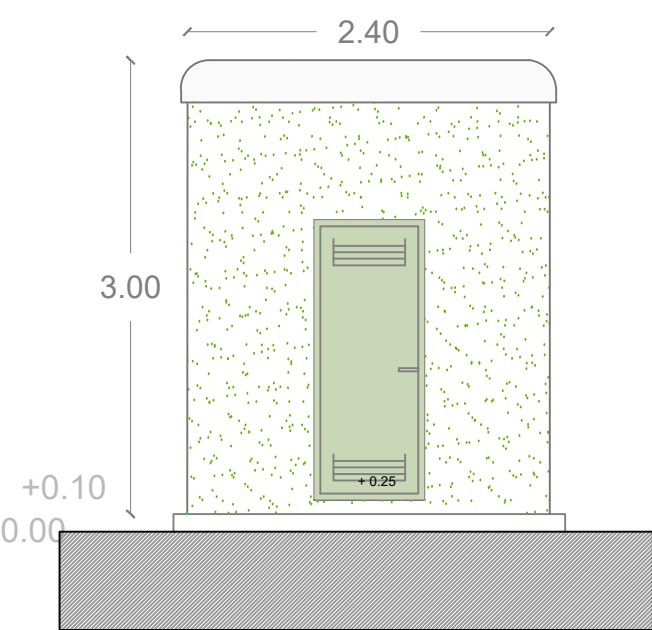
VISTA FRONTALE
