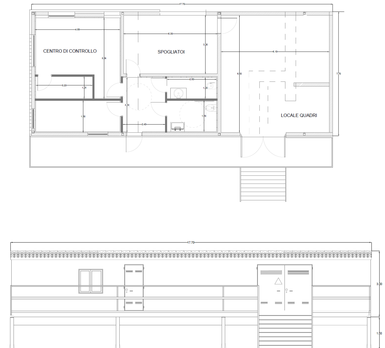
Figura3–Cabina di raccolta e servizi ausiliari
