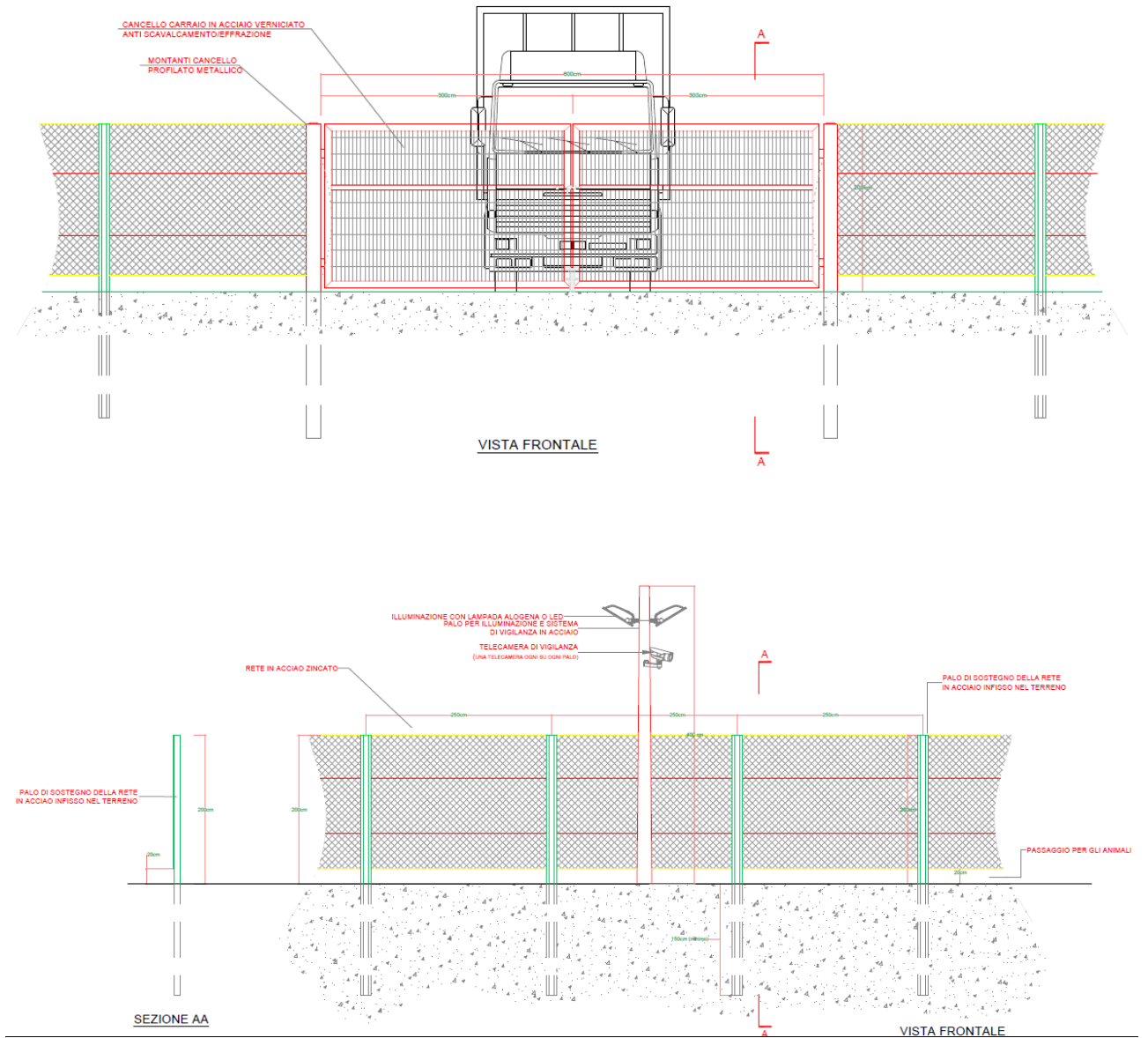
Figura 4–Particolari recinzione e cancello di accesso
