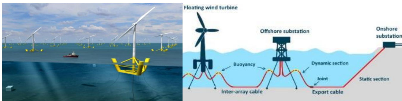
Figura 6 - Struttura di galleggiamento della turbina
