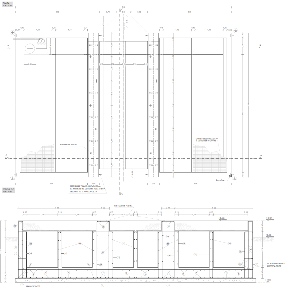
Fig. Pianta e sezione Trasformatore di potenza 150 kV
