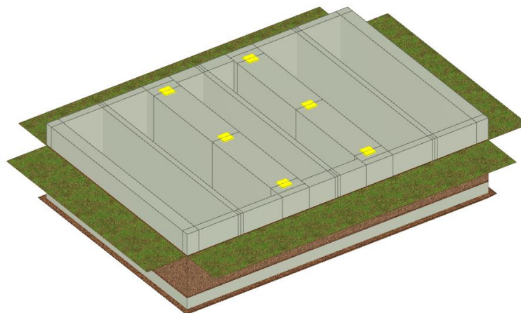
Fig. Vista assonometrica fondazione per trasformatore di potenza 150kV
