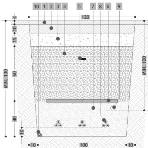
Figura 2: Sezione tipo cavidotto composta da tre terne da 630 mm 2
