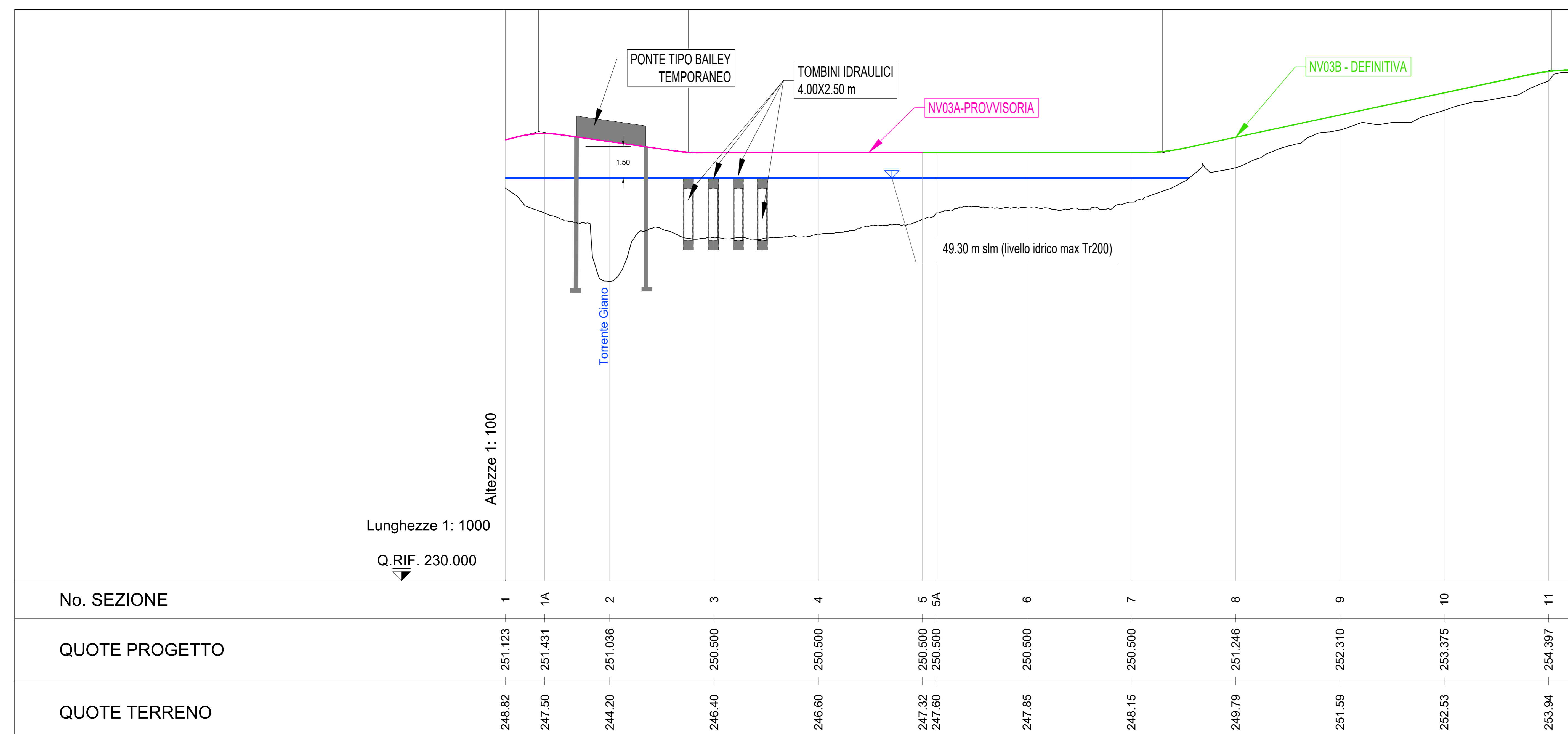
PROFILO LONGITUDINALE NV03 CON LIVELLI IDRICI - scala 1:1000/1:100
