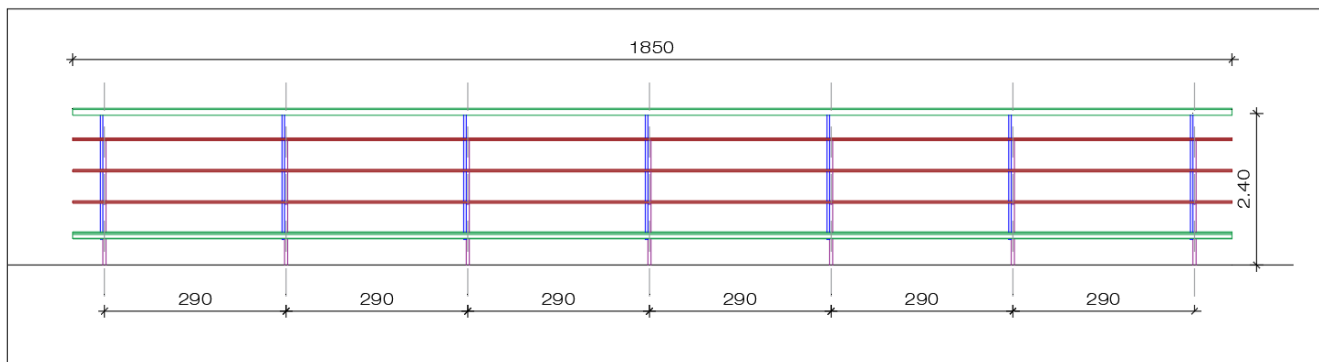
Vista frontale strutture - Modulo 8x4
