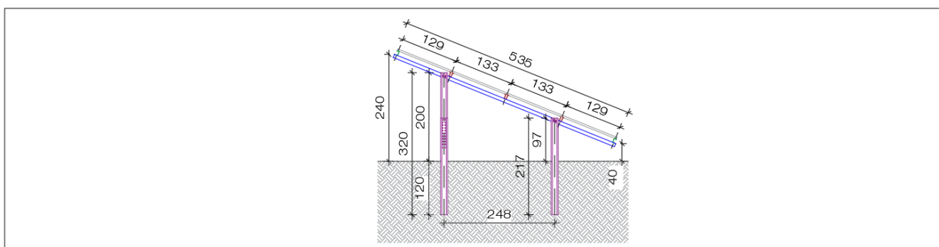
Vista laterale strutture - Modulo 8x4
