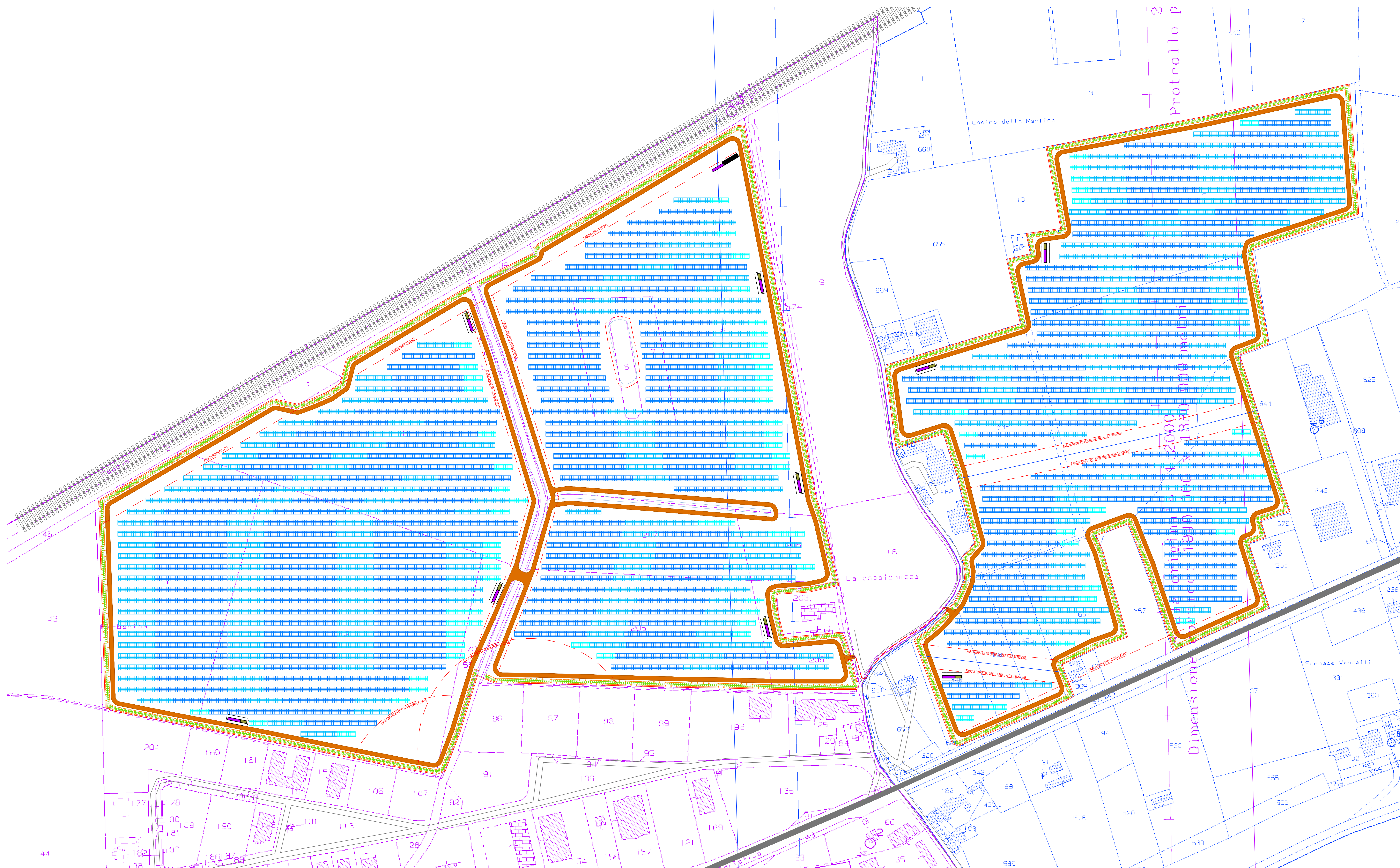
LAYOUT IMPIANTO - CATASTALE Scala 1:1500
